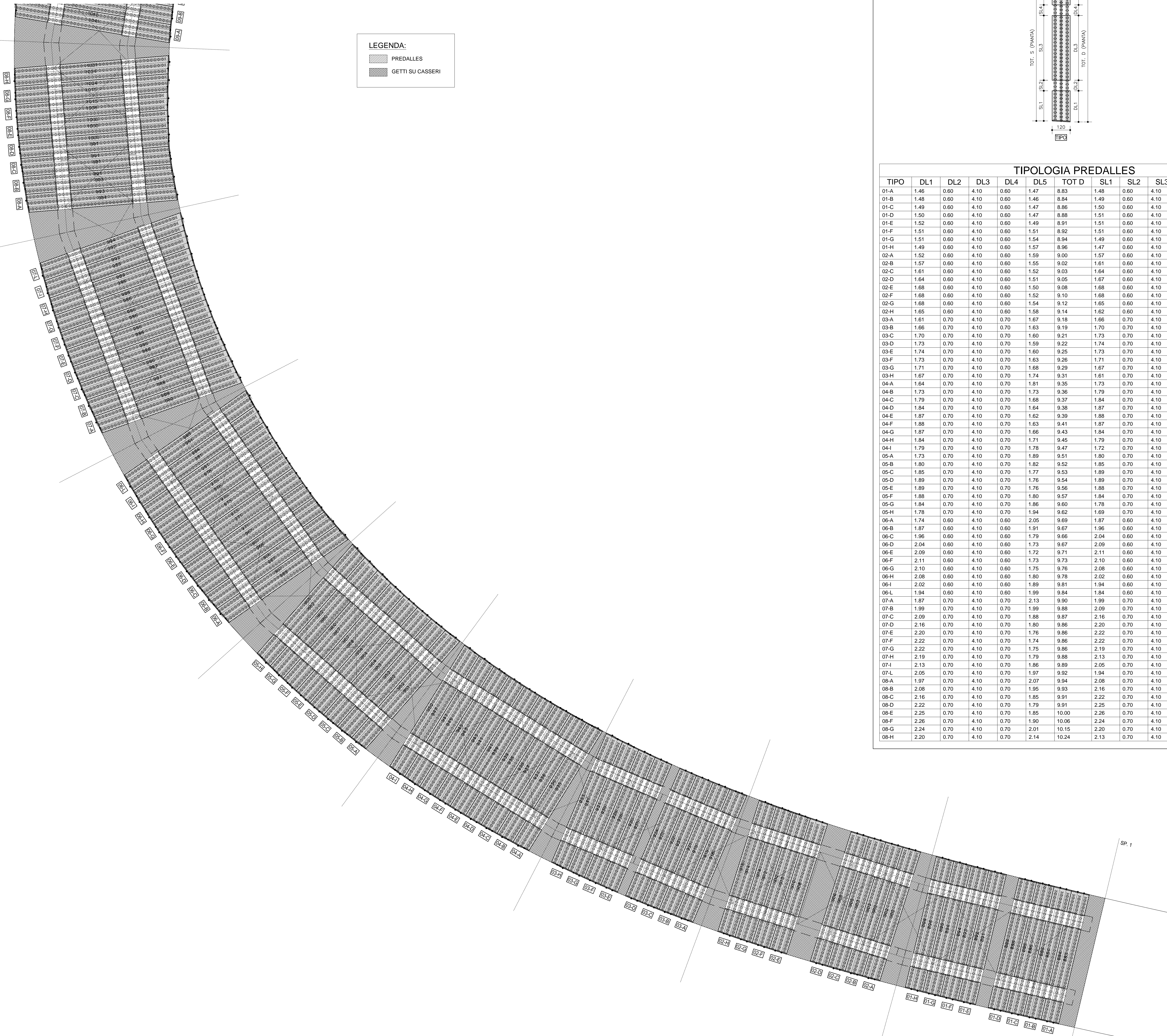
Pianta predalles Viadotto A 1/2 Scala 1:100
