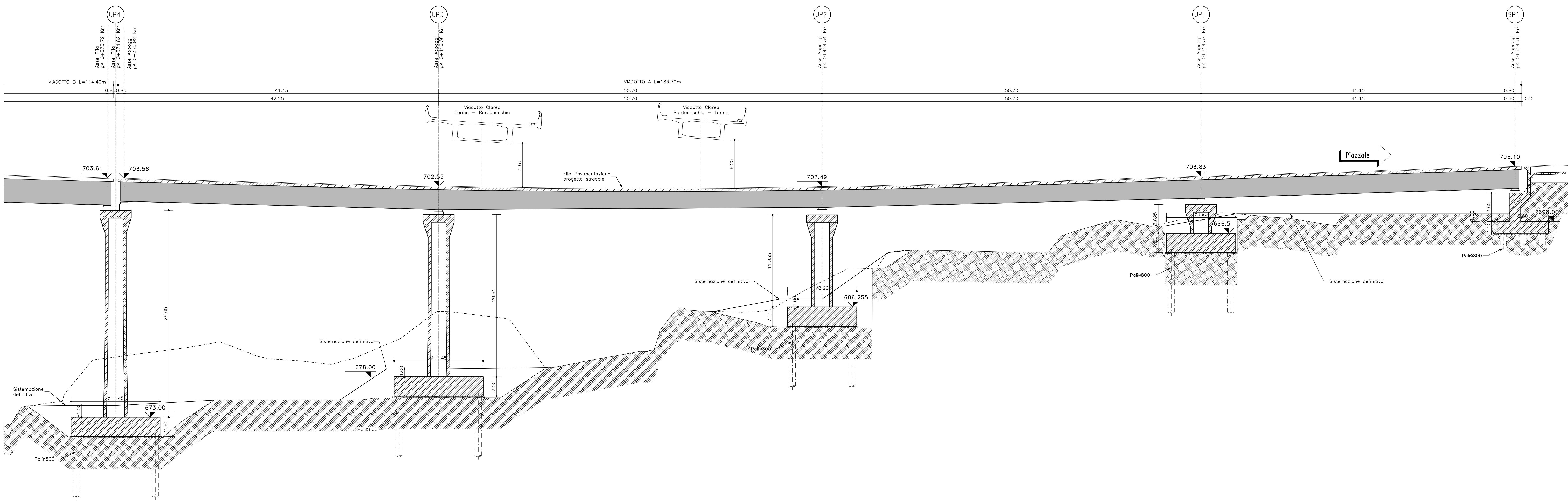
Profilo longitudinale Viadotto A Scala 1:200
