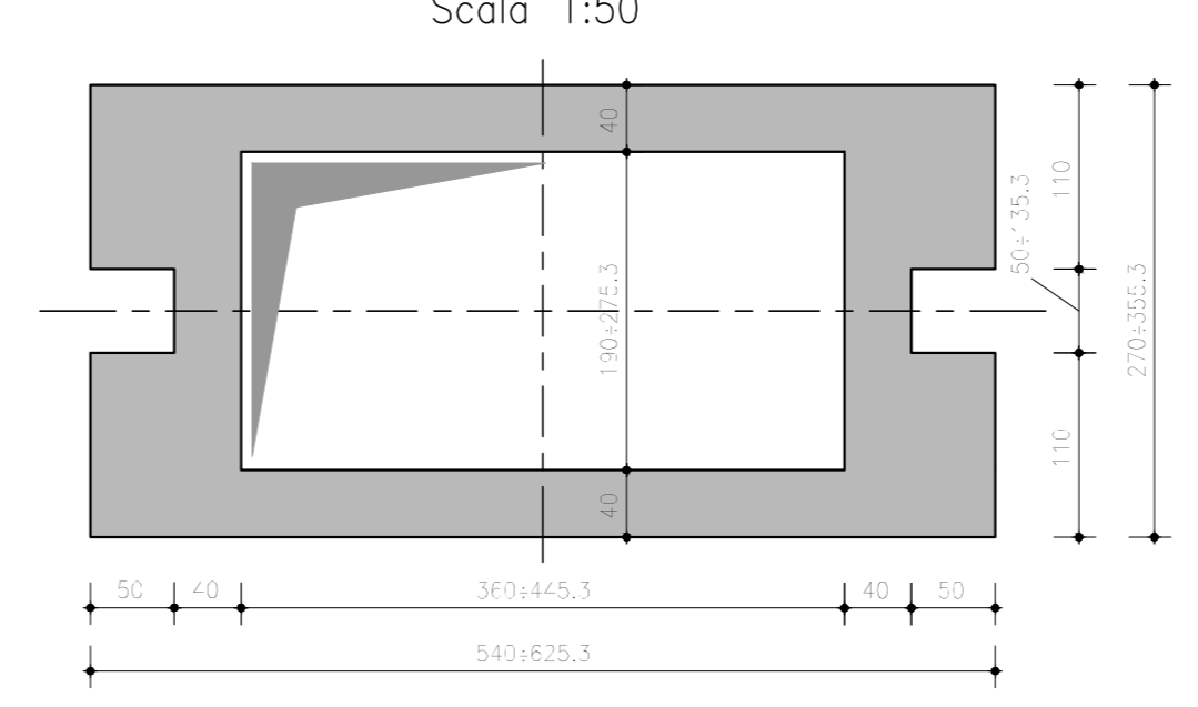
Sezione "C - C" Scala 1:50
