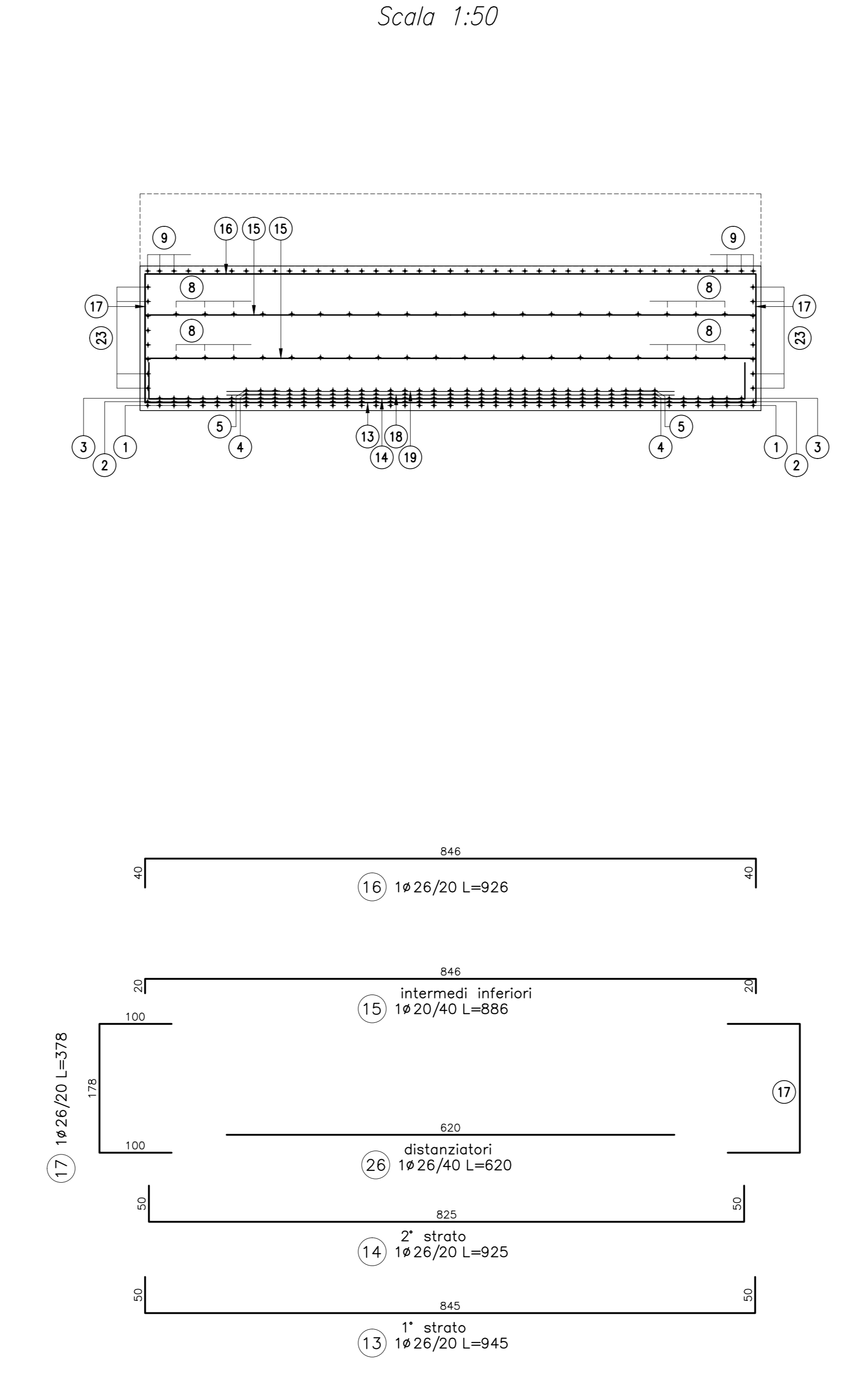
Sezione B-B Scala 1:50
