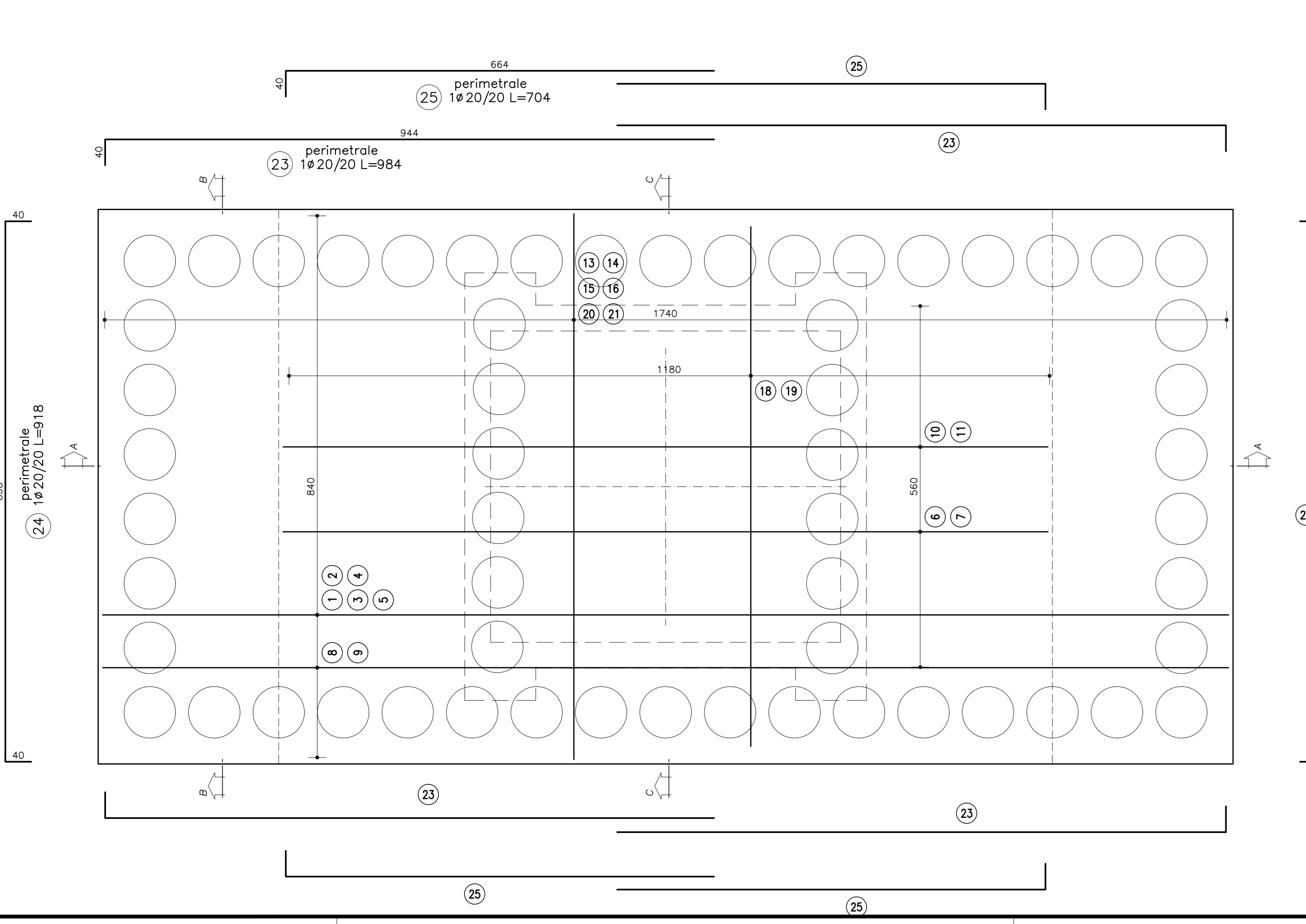
Pianta Scala 1:50
