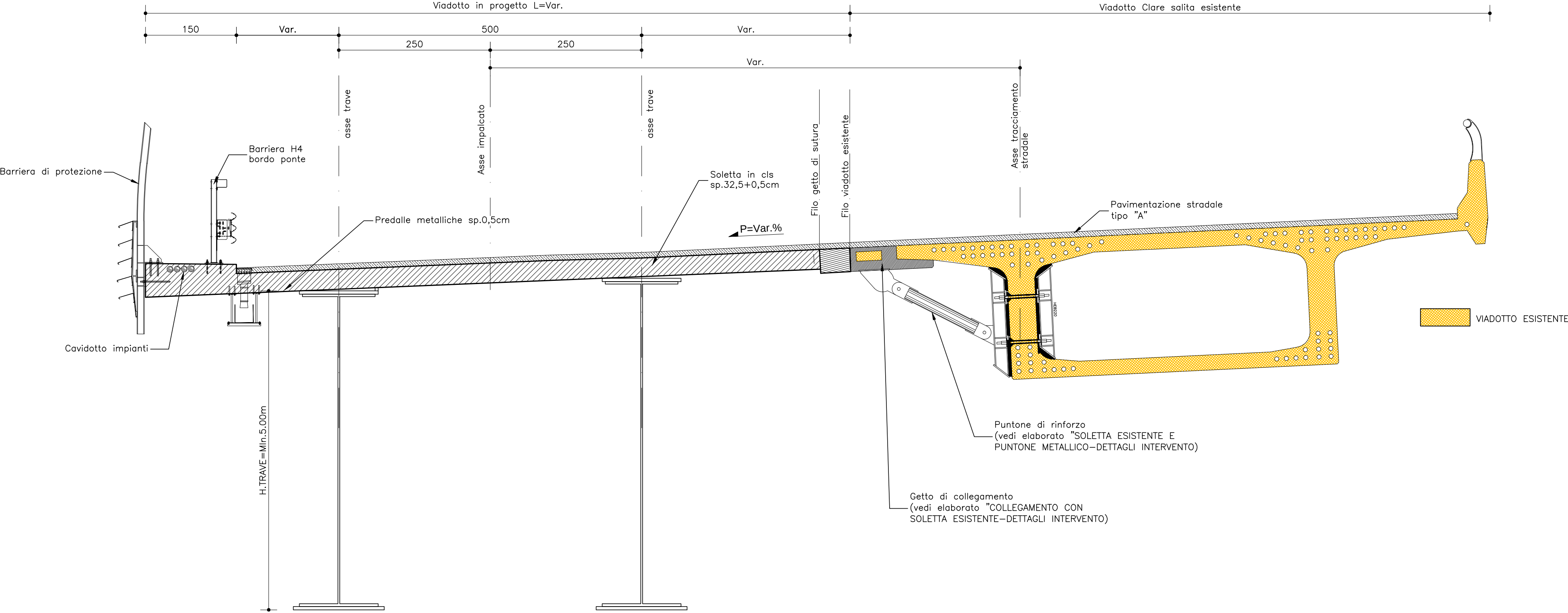
Sezione "C" impalcato in campata (da UP7 a fine viadotto) Scala 1:50
