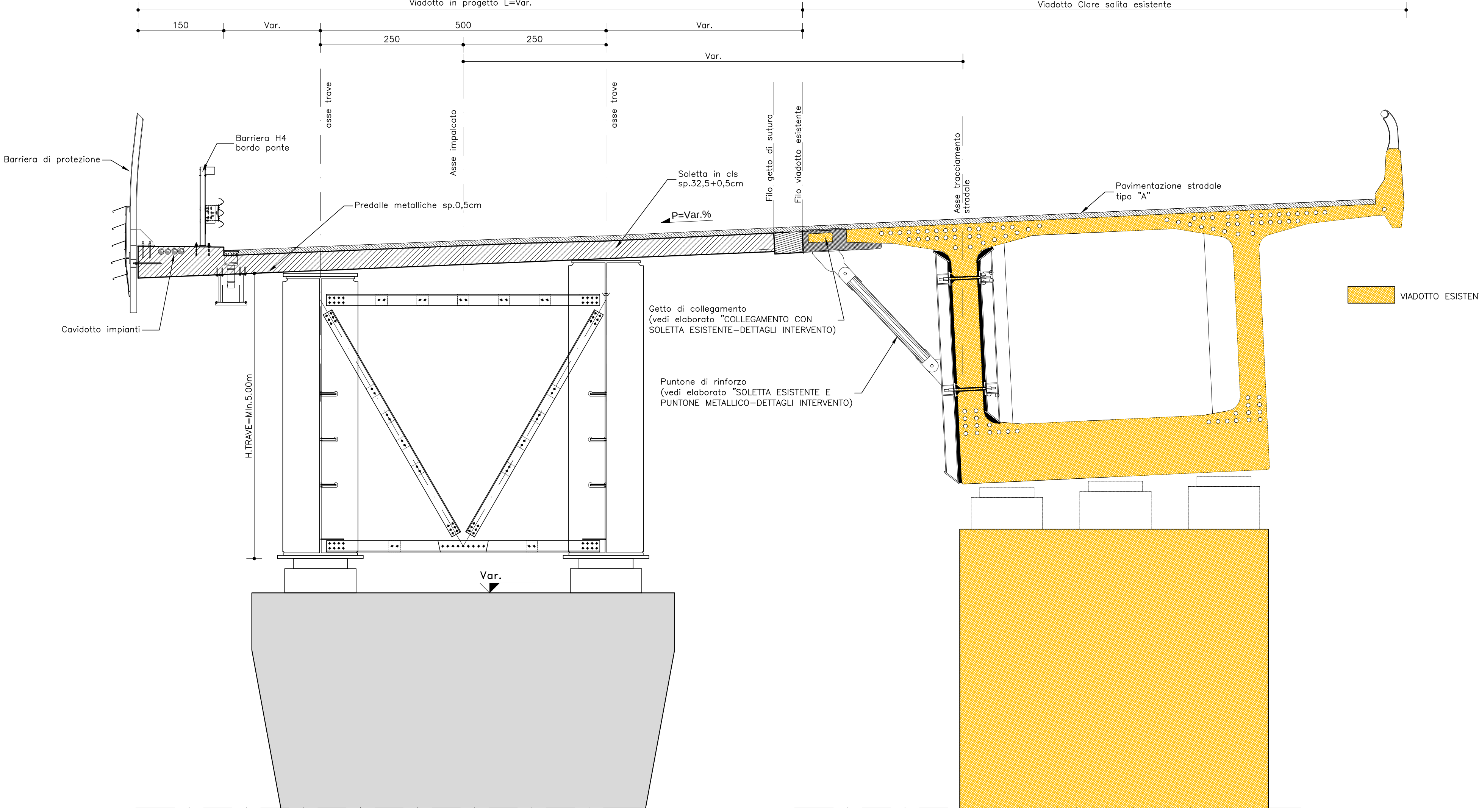
Sezione "D" impalcato su PILA UP 7 - UP 9 Scala 1:50
