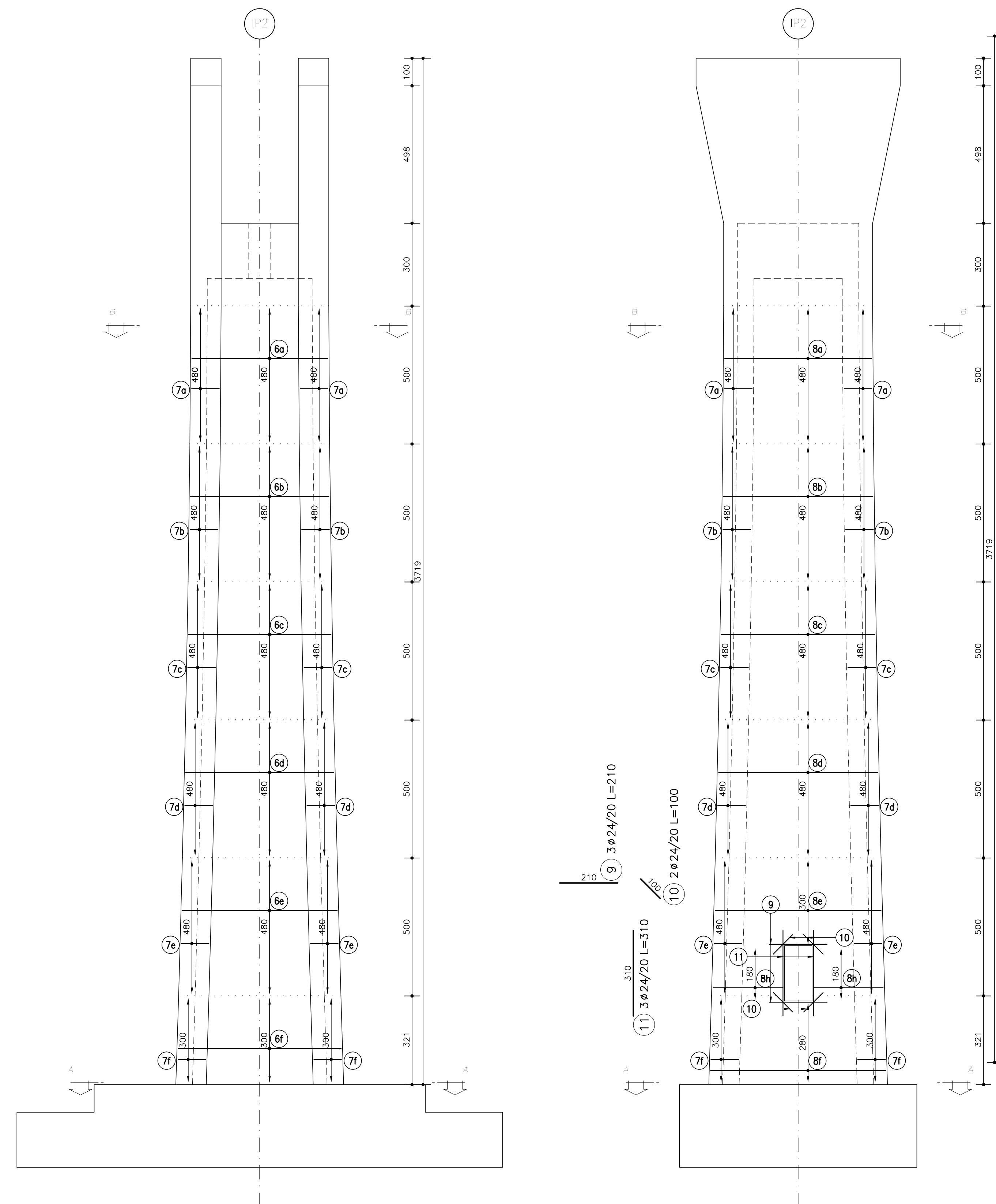
Armatura orizzontale Scala 1:100
