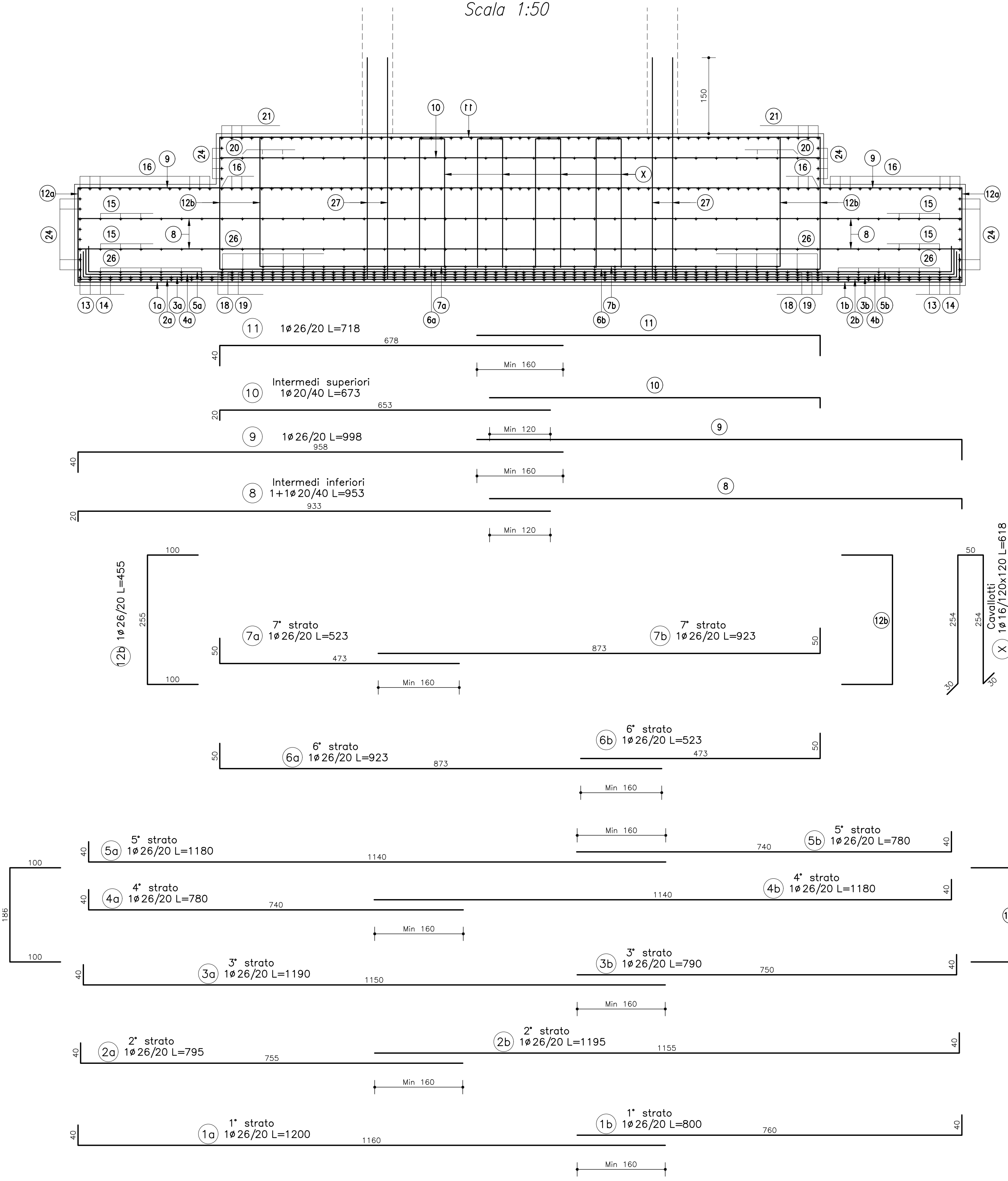
Sezione A-A Scala 1:50
