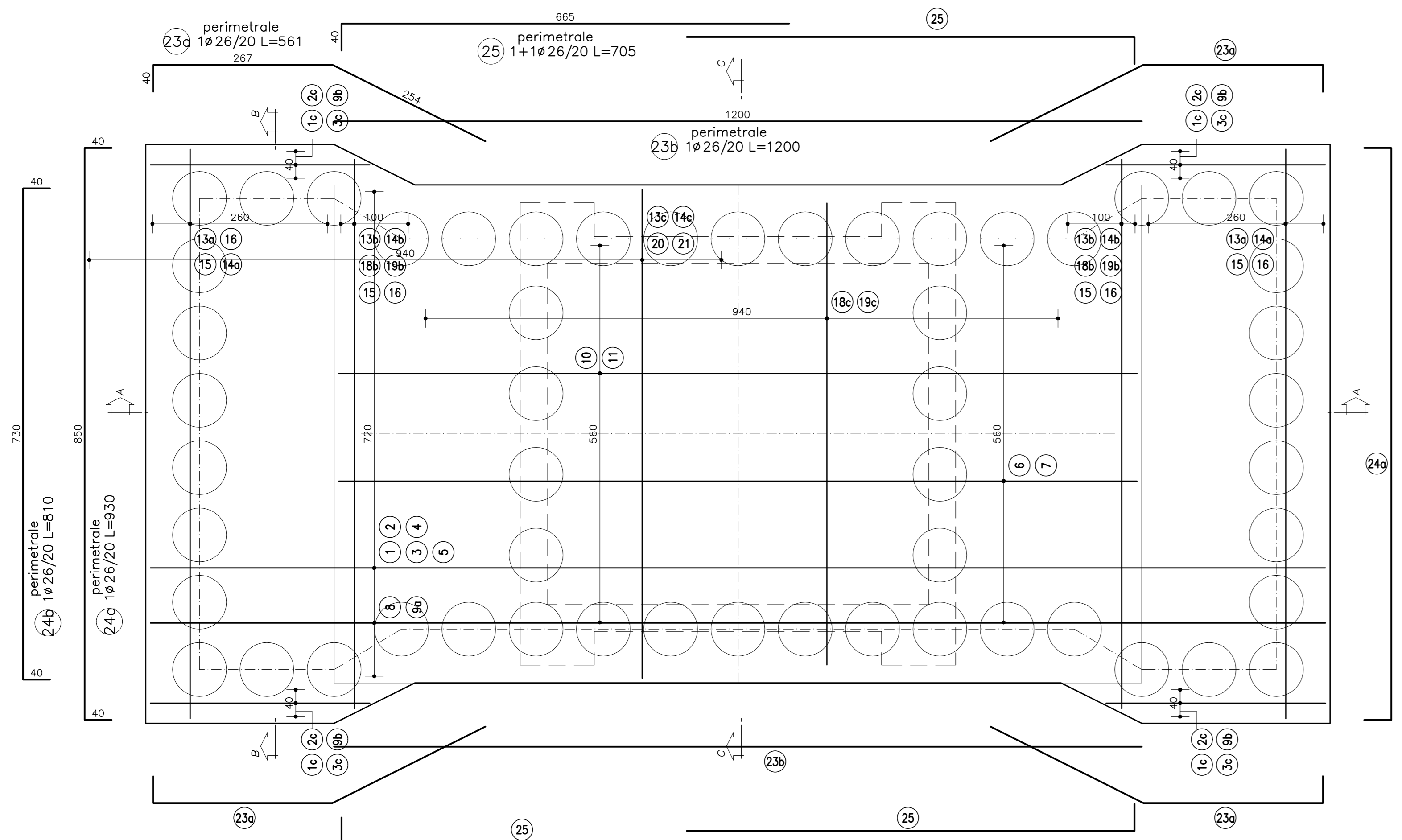
Pianta Scala 1:50
