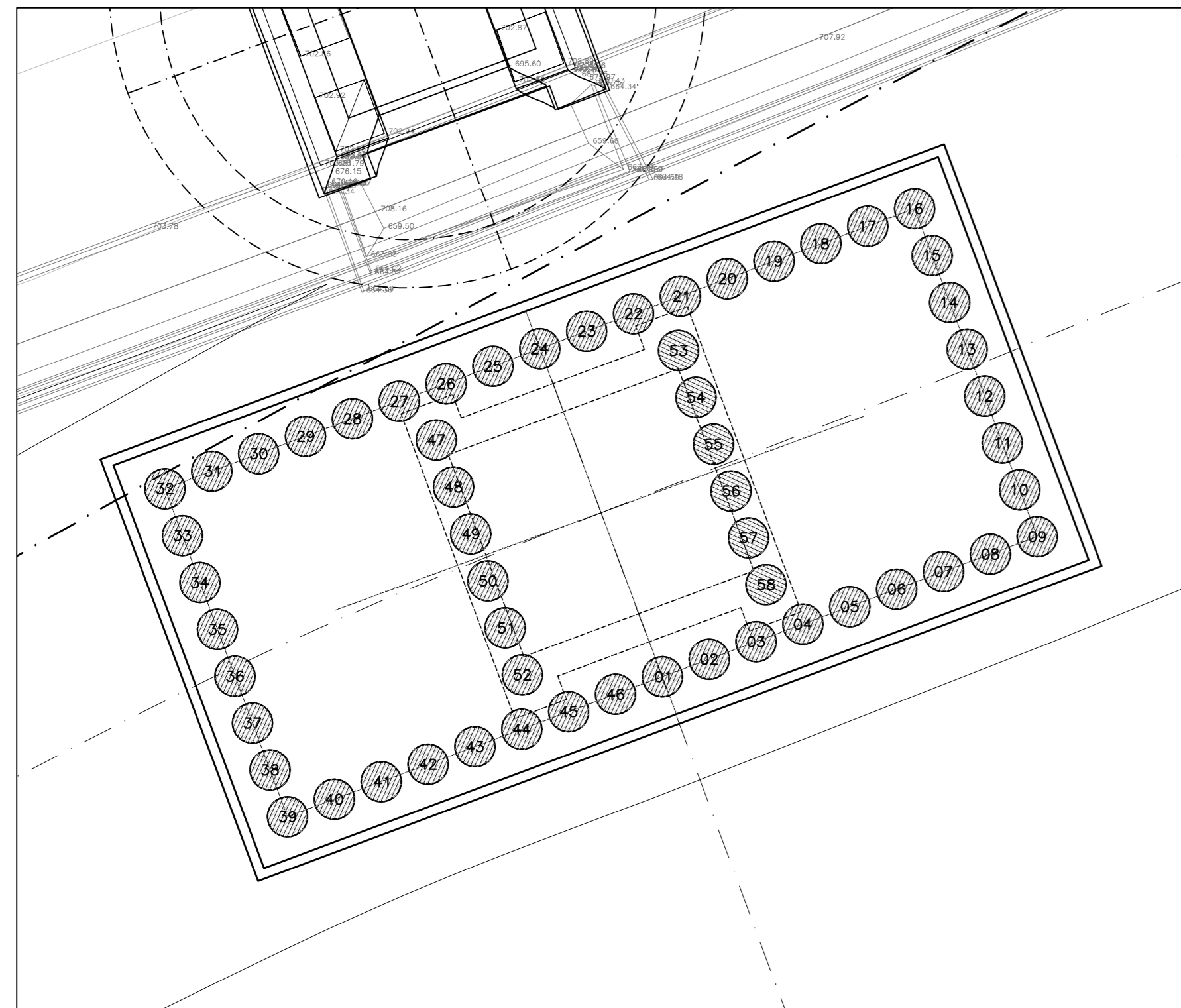
Pila IP2 Scala 1:100
