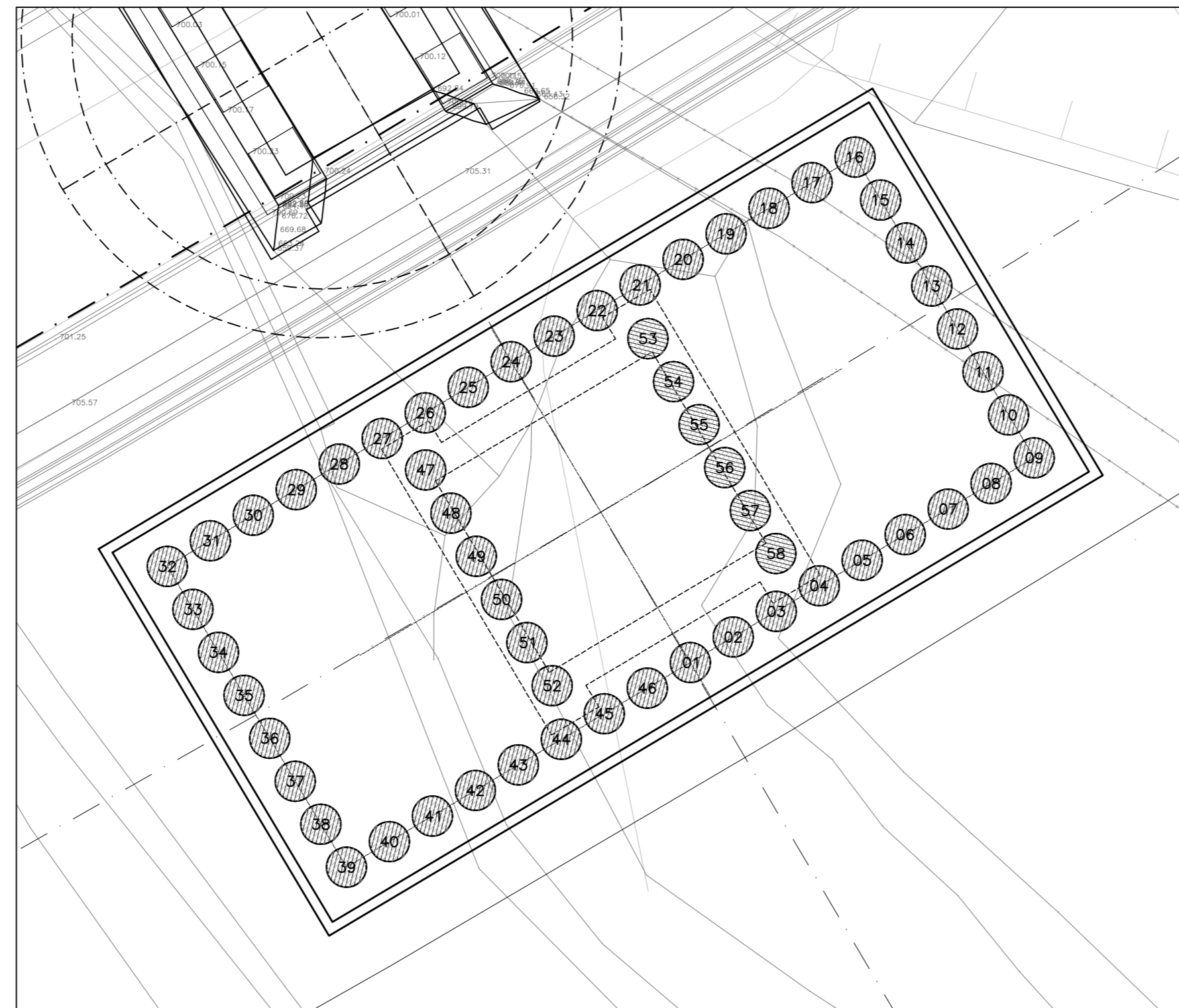
Pila IP3 Scala 1:100
