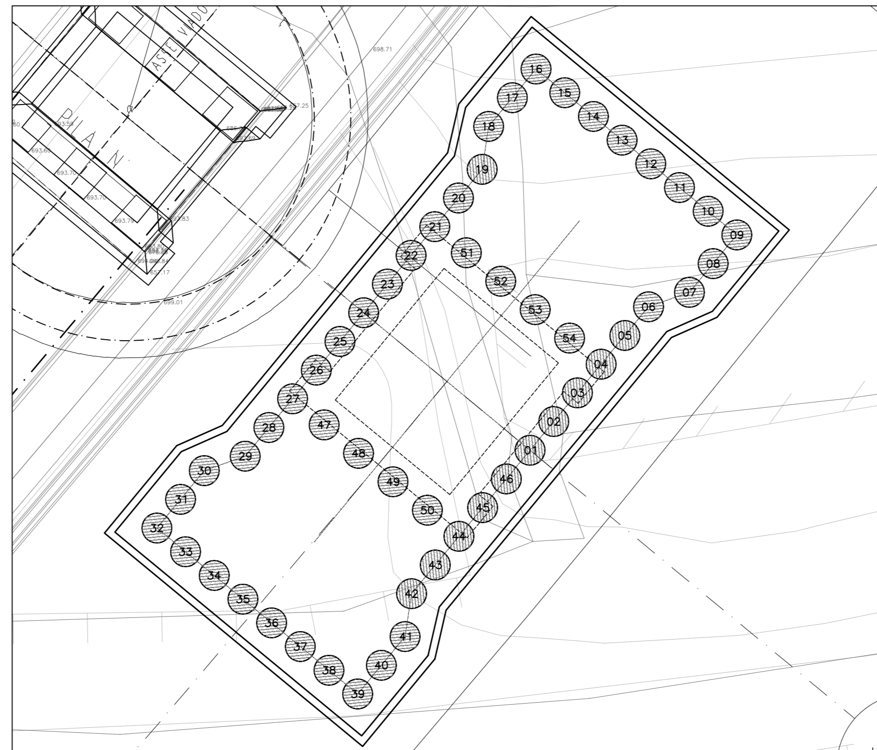
Pila IP5 Scala 1:100
