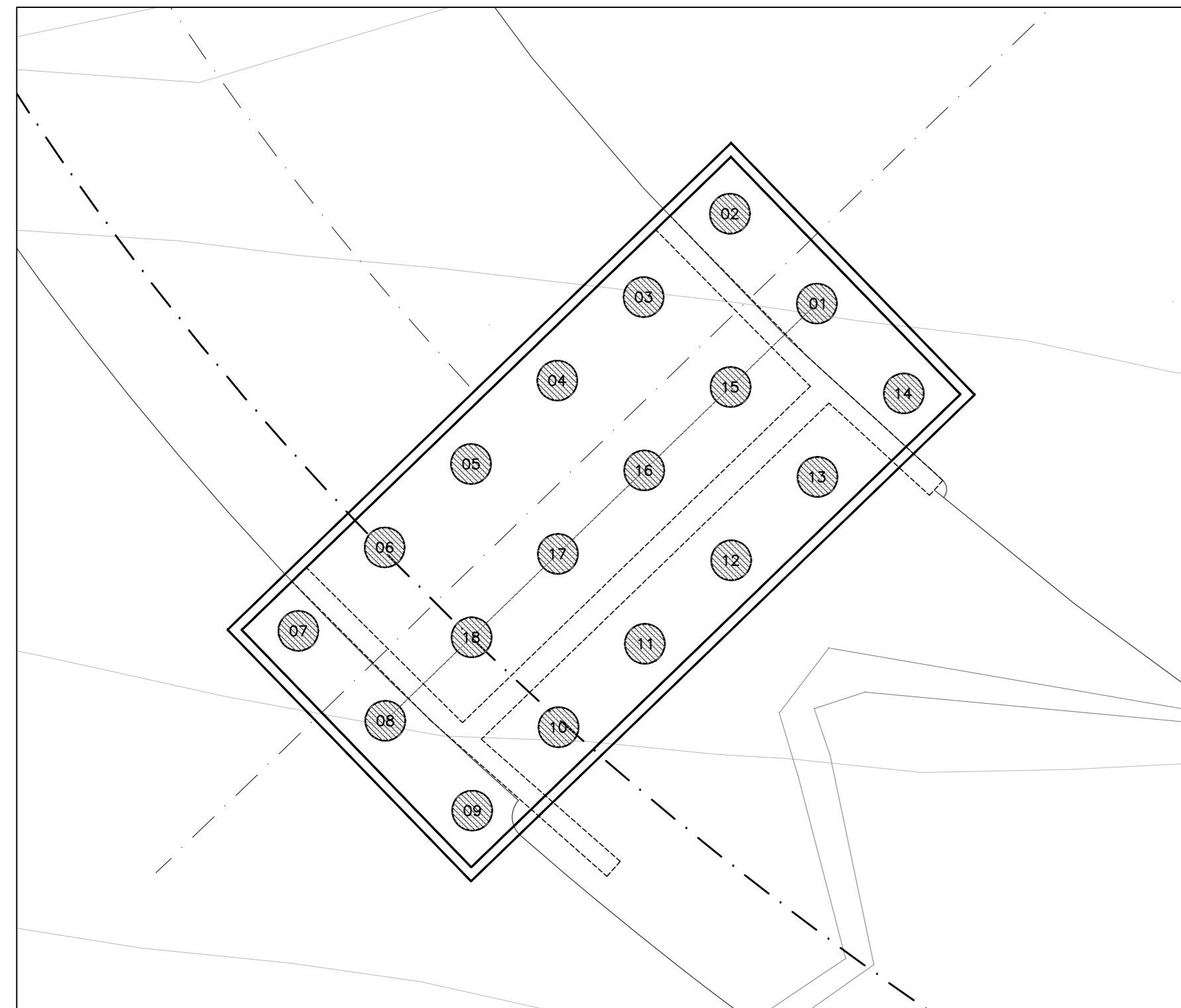
Spalla SP2 Scala 1:100
