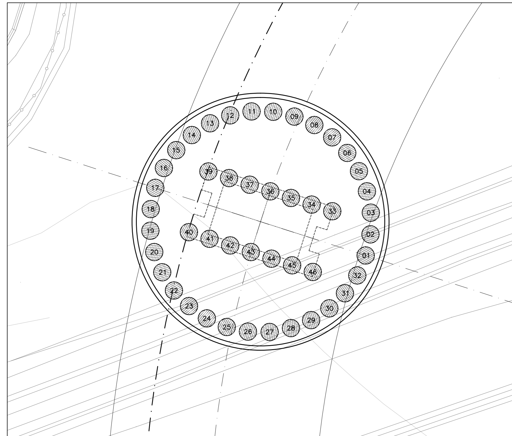
Pila IP1 Scala 1:100
