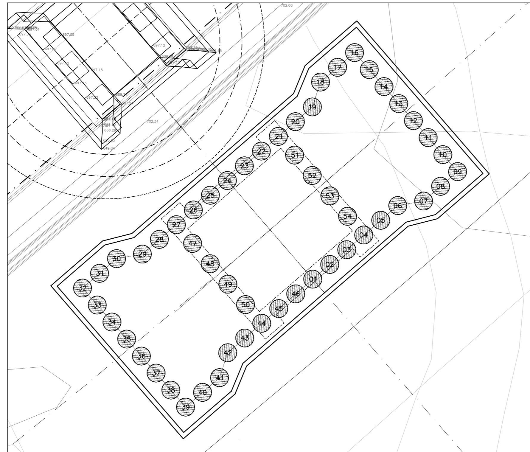
Pila IP4 Scala 1:100
