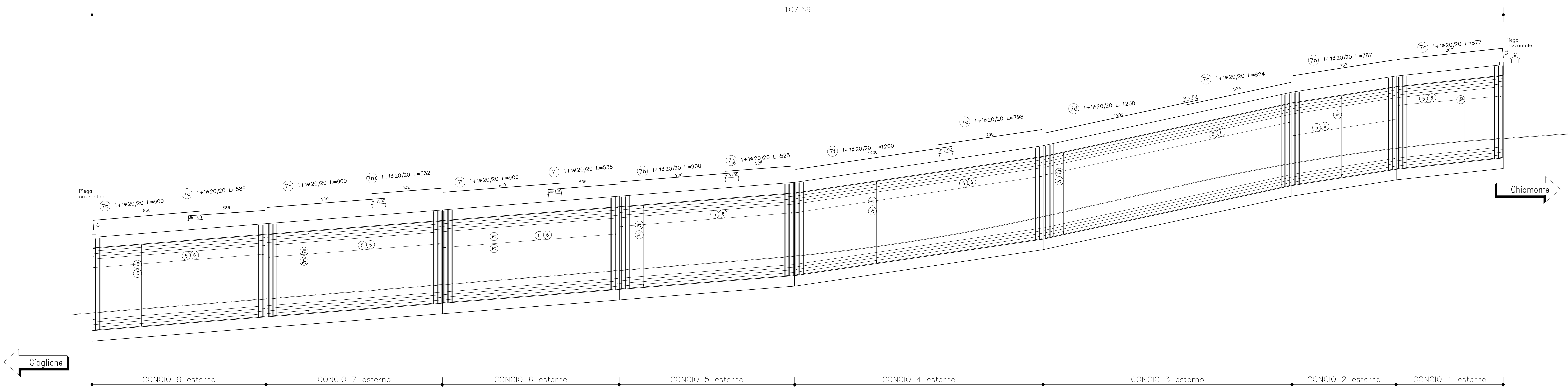
SVILUPPATA B-B Scala 1:100
