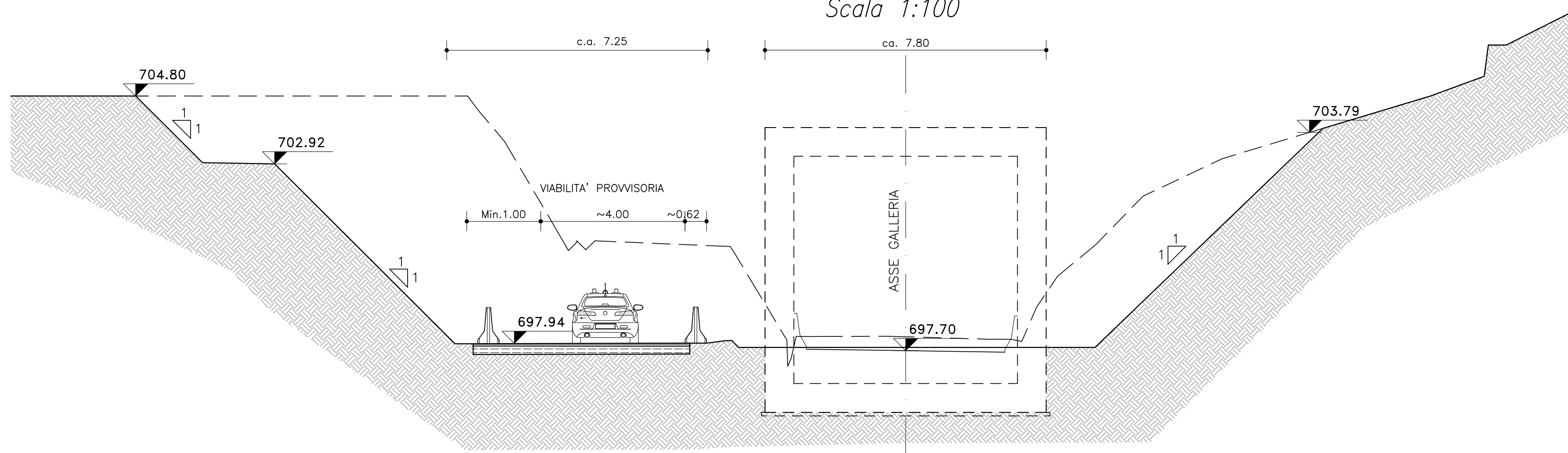
Sezione B-B Scala 1:100
