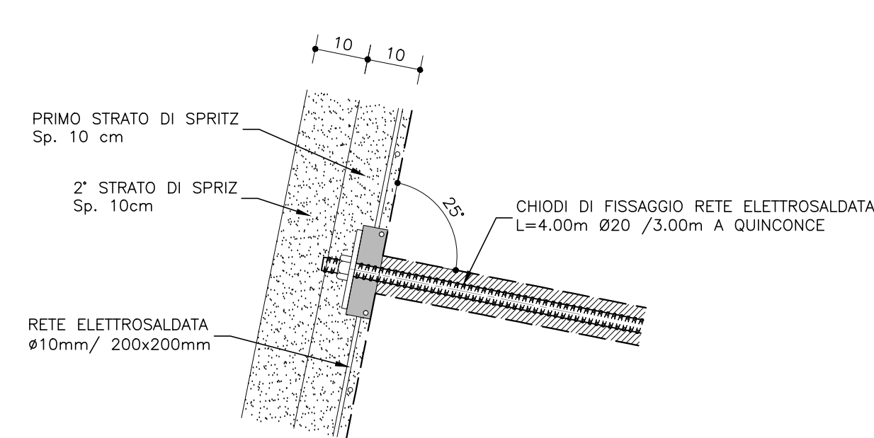
Particolare spritz beton a protezione dello scavo Scala 1:10
