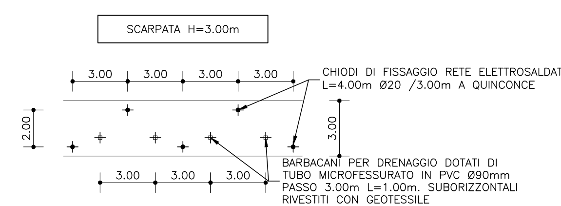
Particolare posizionamento chiodi e drenaggi Scala 1:200
