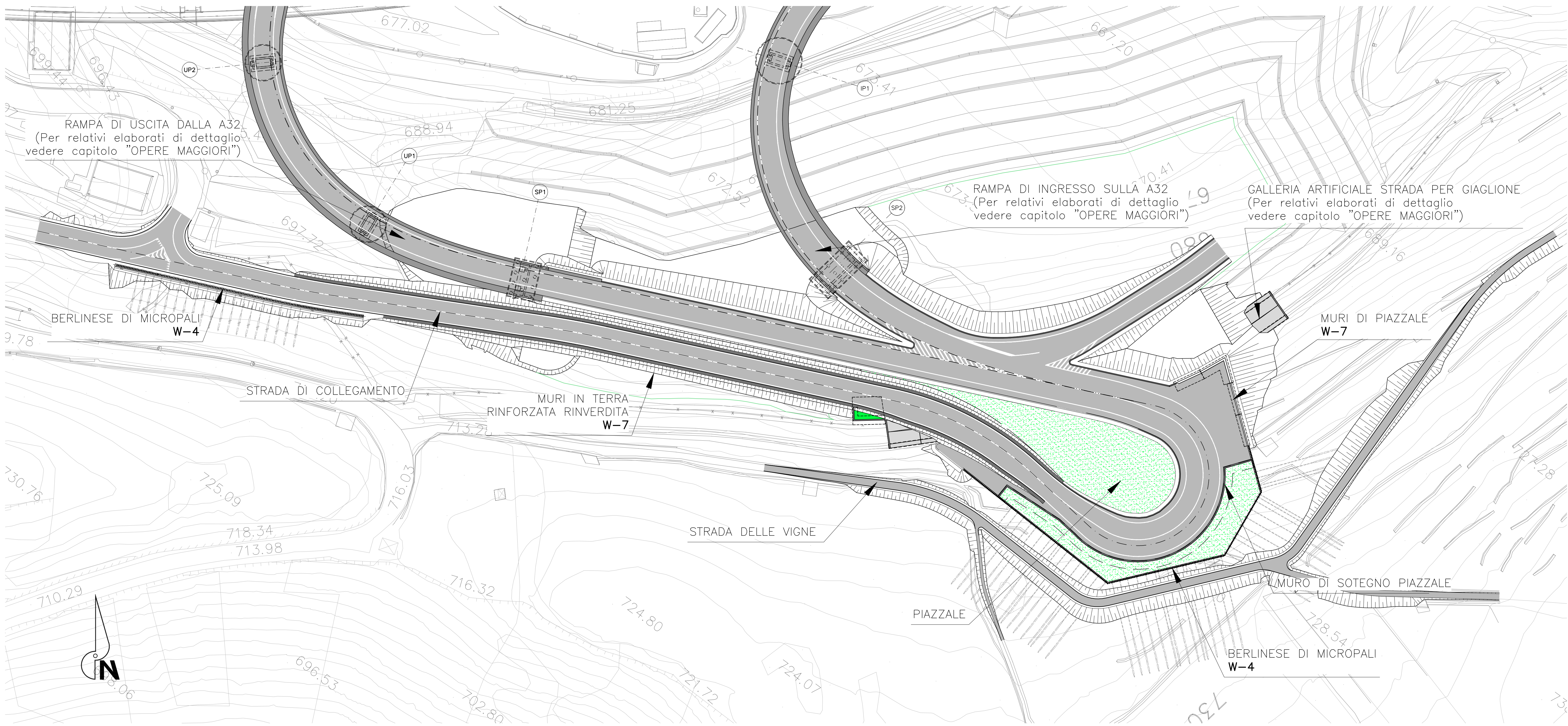
PIANTA Scala 1:500
