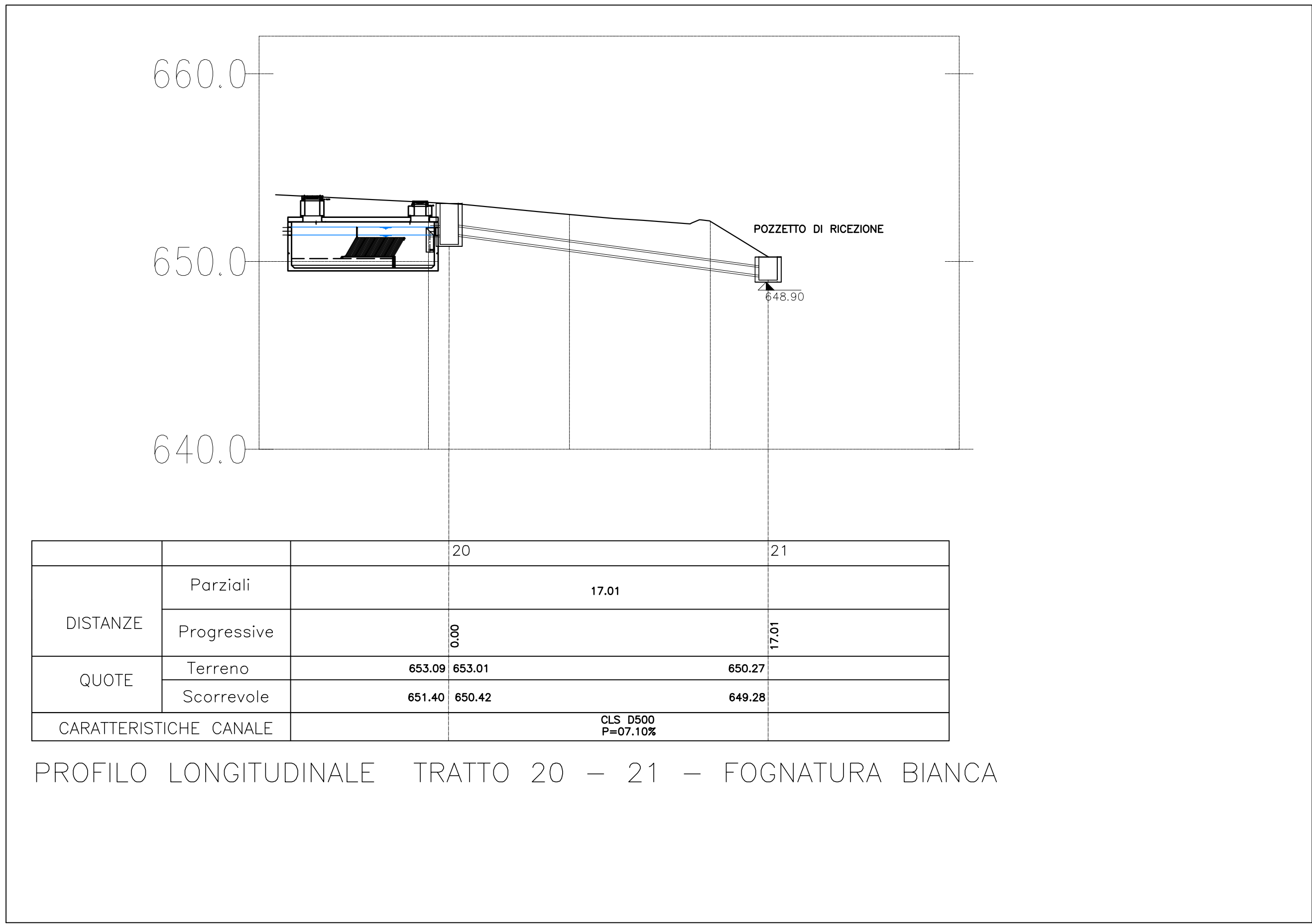
PROFILO LONGITUDINALE SECONDO TRATTO TUBAZIONE SCALA 1:200
