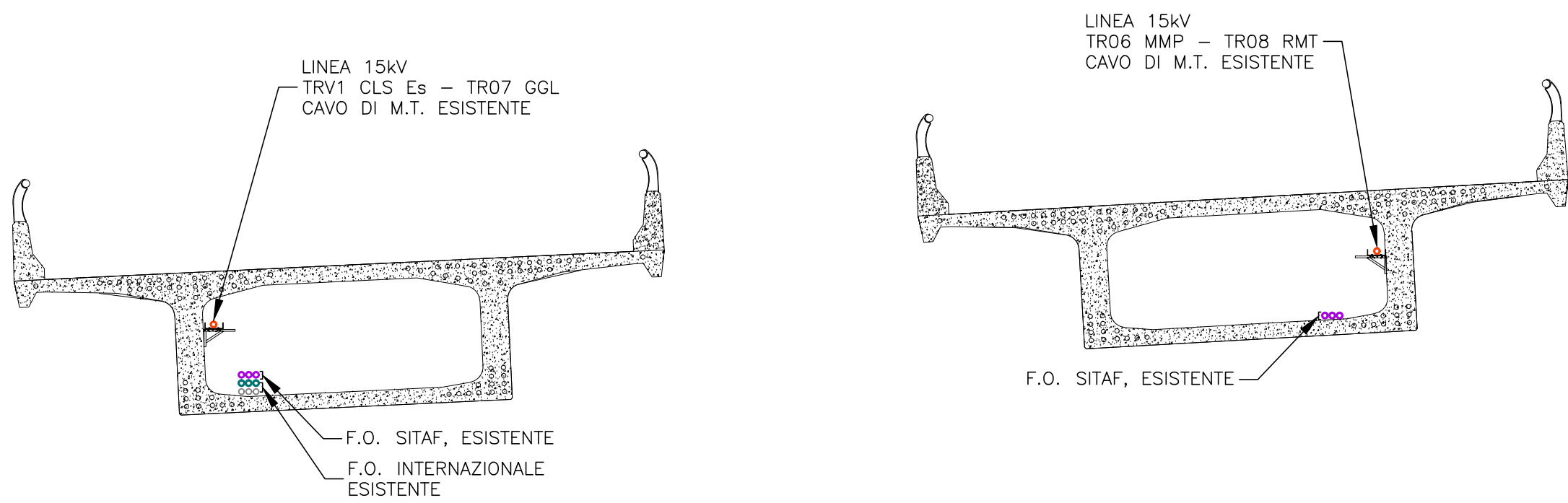
SEZIONE TRASVERSALE A-A AUTOSTRADA A32 Scala 1:100
