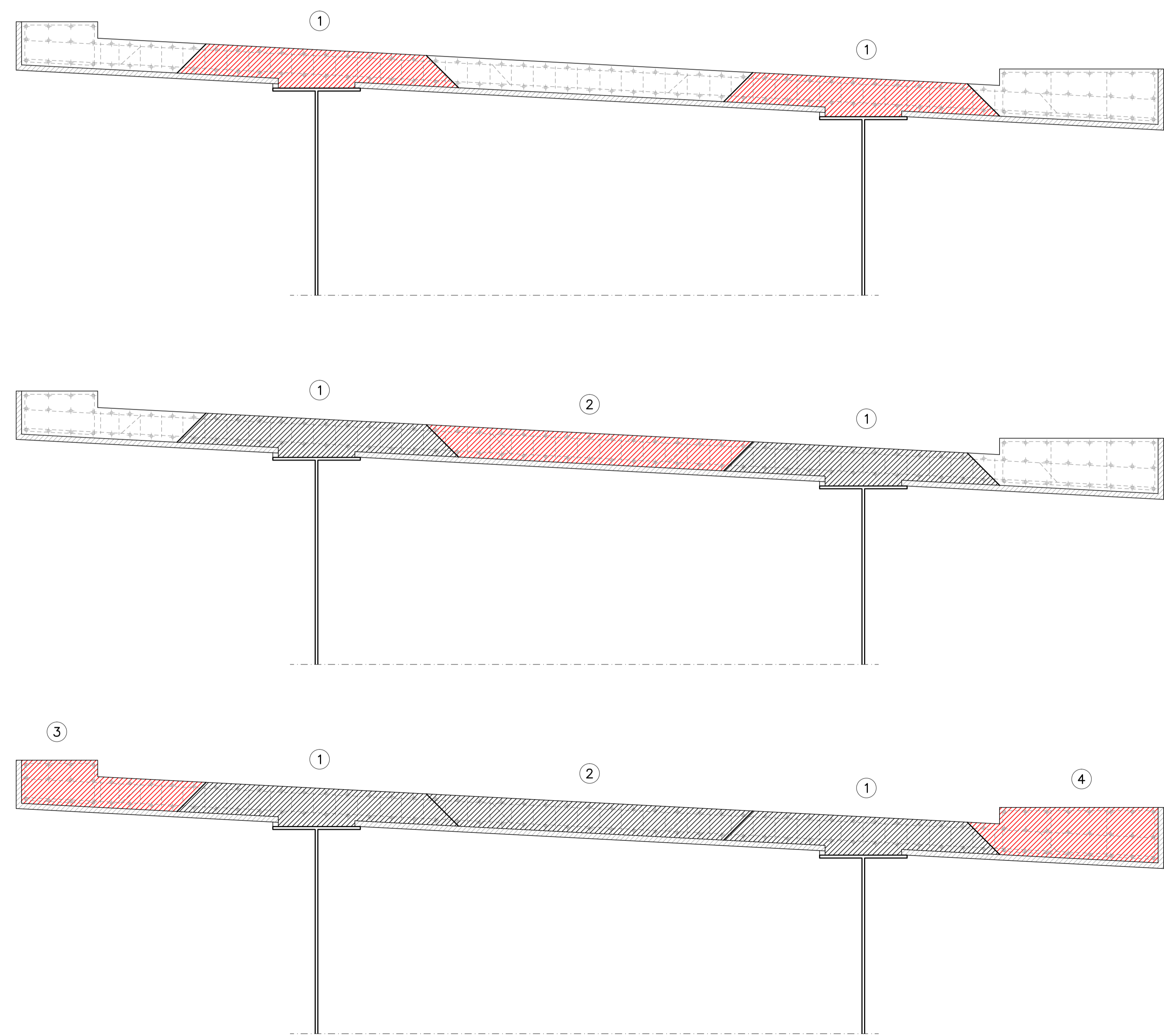
Sezione Tipo - Fasi di getto - Scala 1:50
