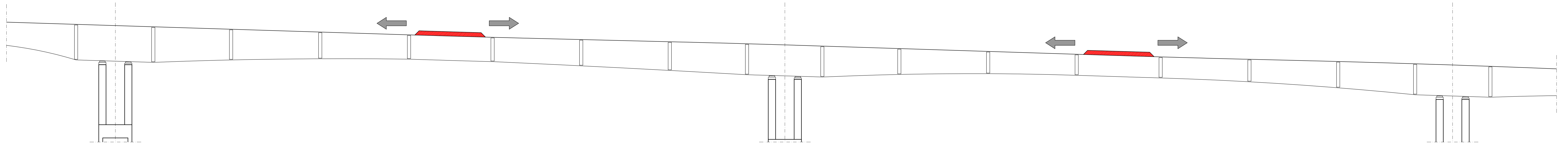
Profilo longitudinale campata Tipo - Fasi di getto - Scala 1:200
