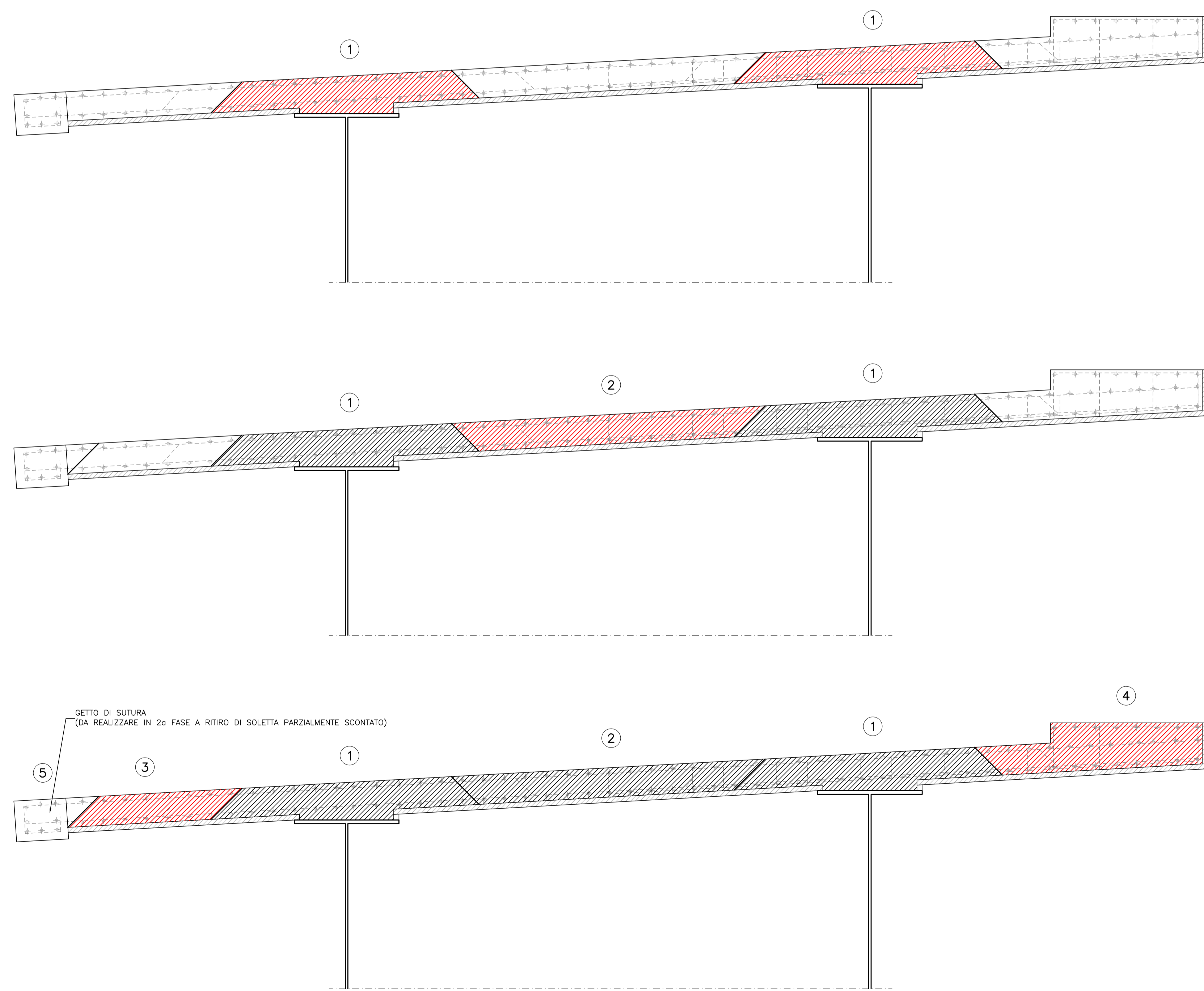
Sezione in affiancamento - Fasi di getto - Scala 1:50
