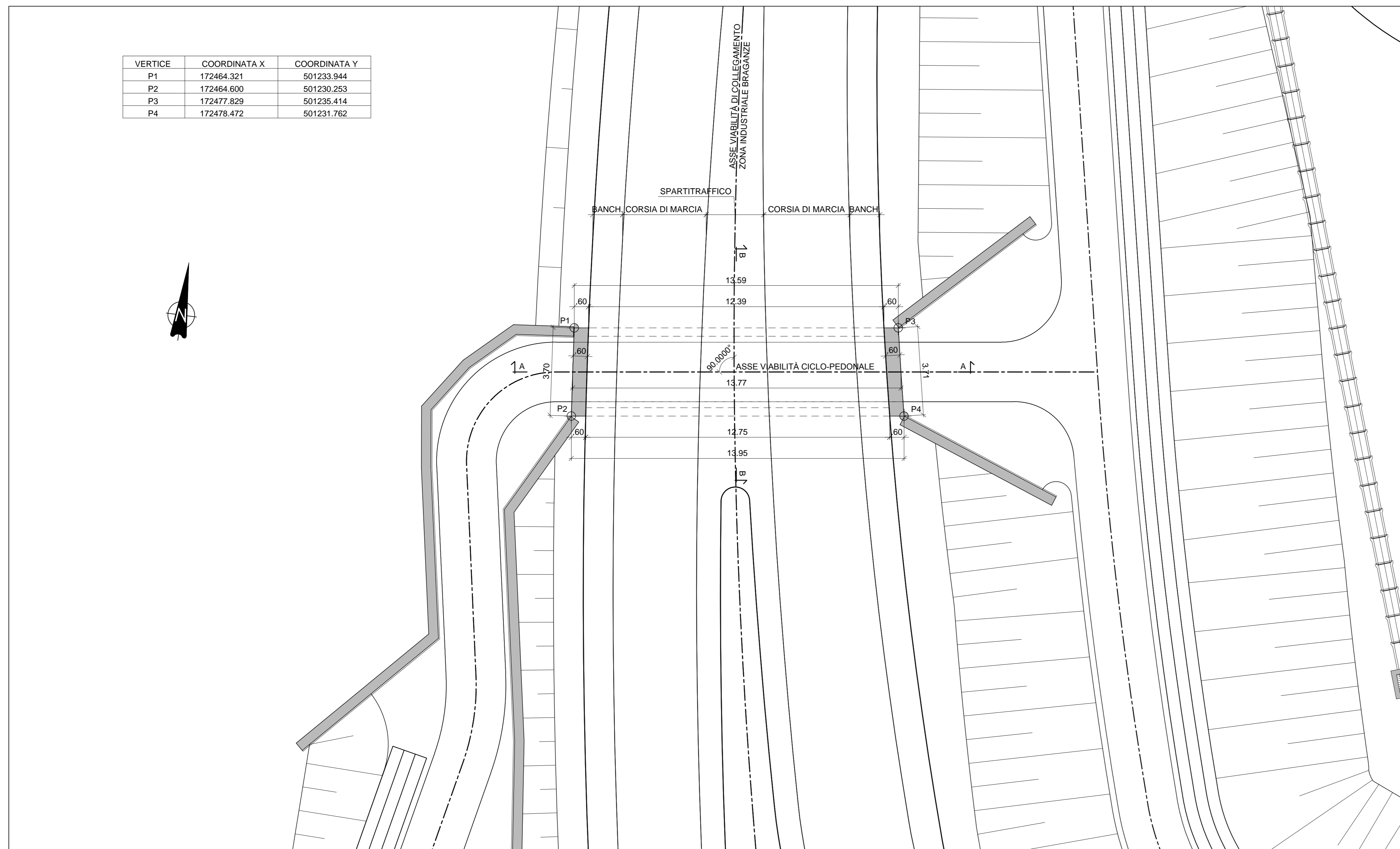
PIANTA QUOTA STRADA INFERIORE - SCALA 1:100
