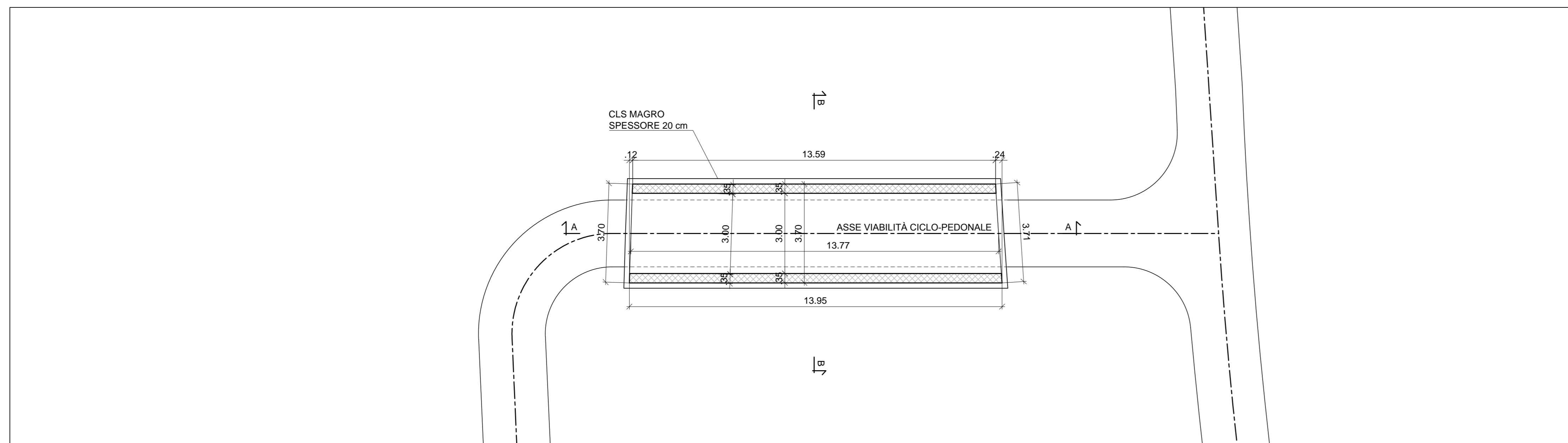
PIANTA QUOTA STRADA INFERIORE - SCALA 1:100
