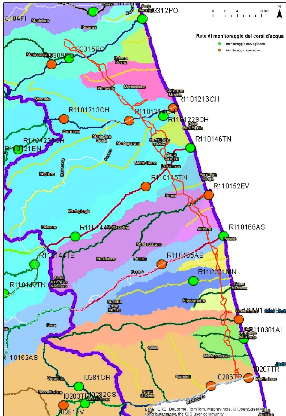
Fig. 6.A: Interazione tra le linee dei metanodotti in progetto e dismissione (linee in rosso) e la rete di monitoraggio regionale delle acque superficiali (Immagine scaricata e modificata da http://www.arpa.marche.it/index.php/fiumi/monitoraggio/attivita )
