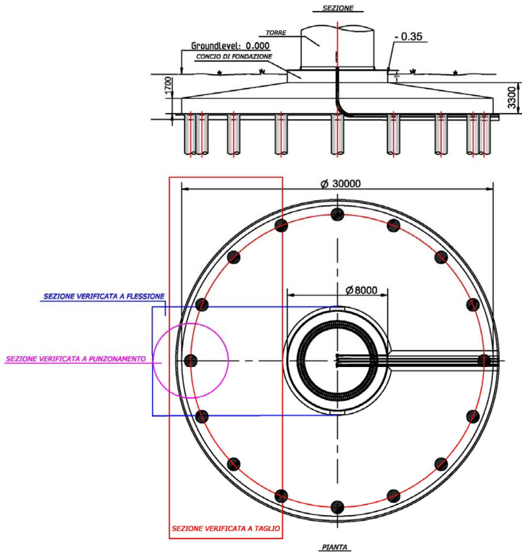
Figura 1 – Fondazione: pianta e sezione
