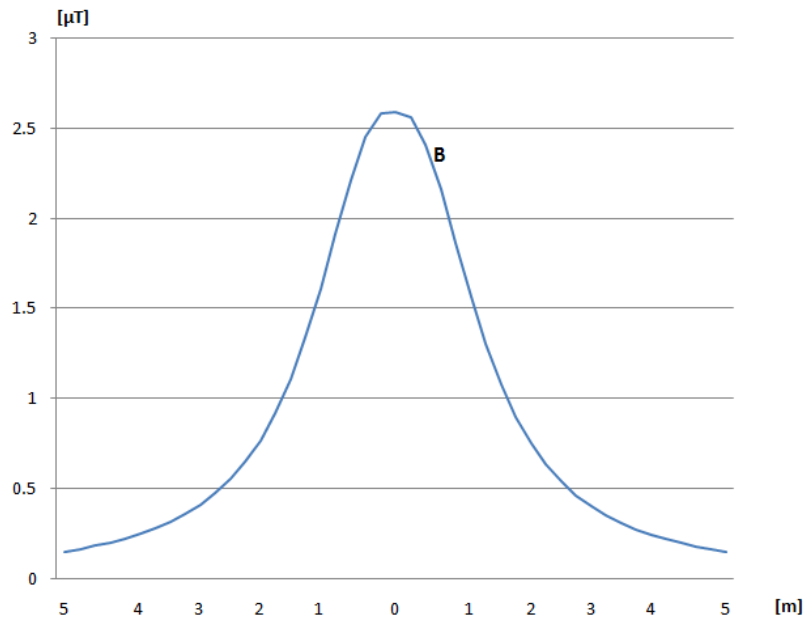
Fig. 5.6 - Campo magnetico generato dagli elettrodotto a 30 kV
