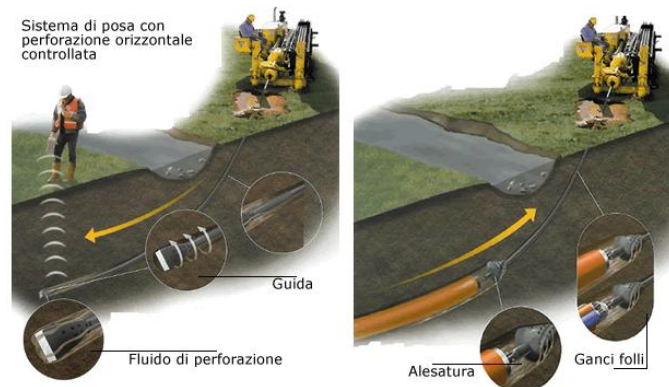
Fig. 1.7 – Posa in opera tubazione per alloggio cavi
