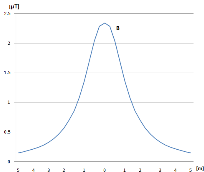
Fig. 2.8 - Campo magnetico generato da elettrodotto interrato a 150kV
