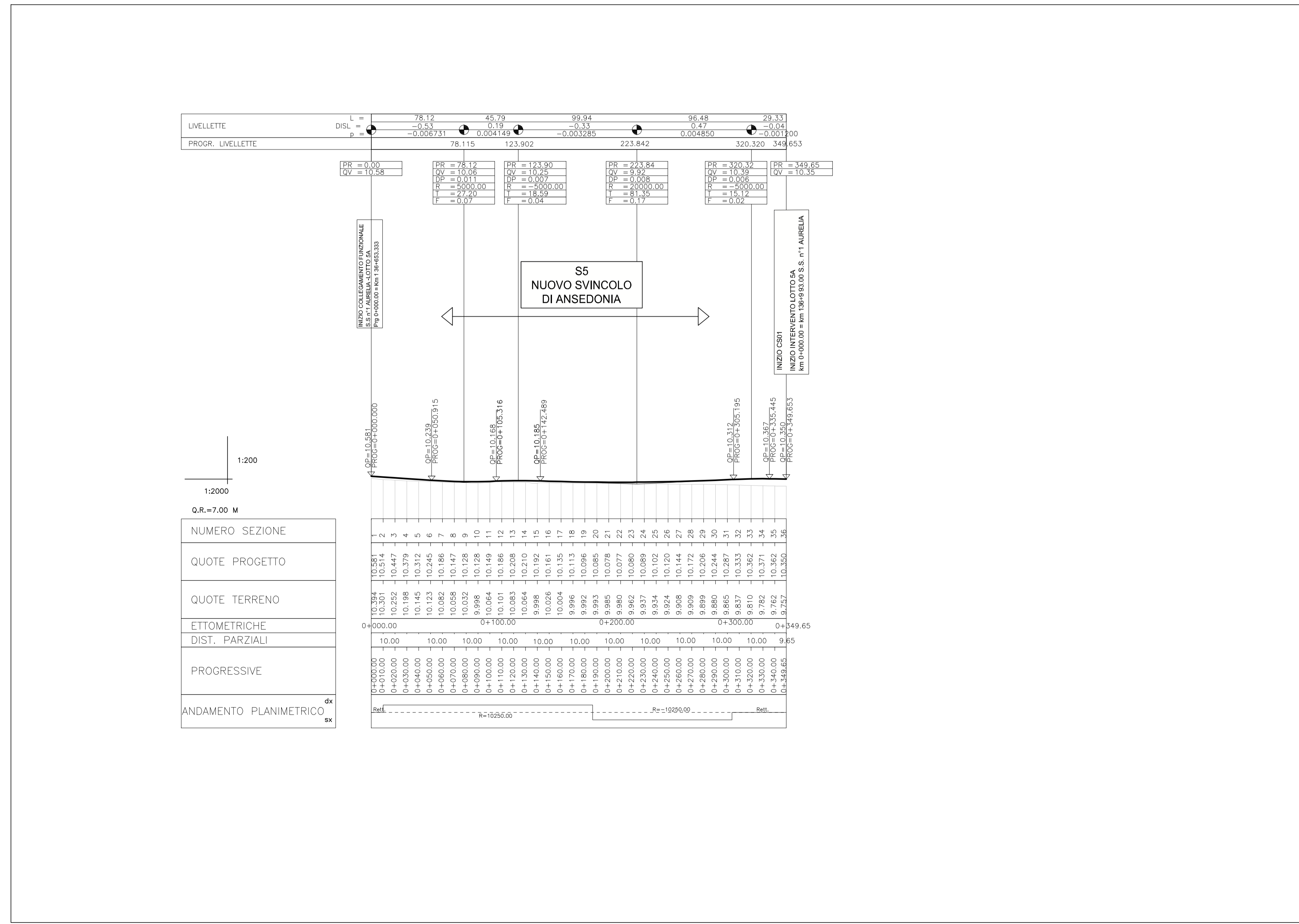
Profilo longitudinale Scala 1:2000/200
