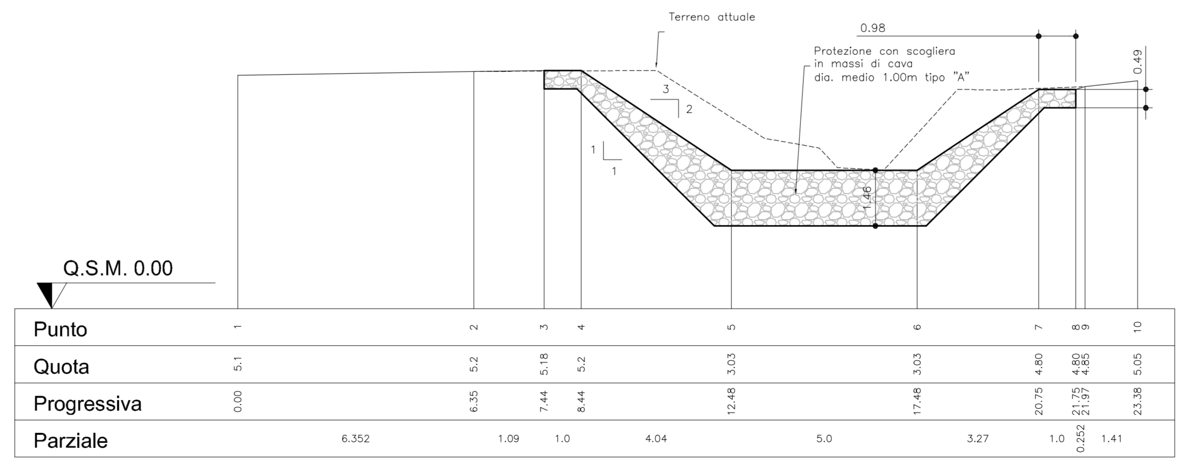
SEZIONE B-B
