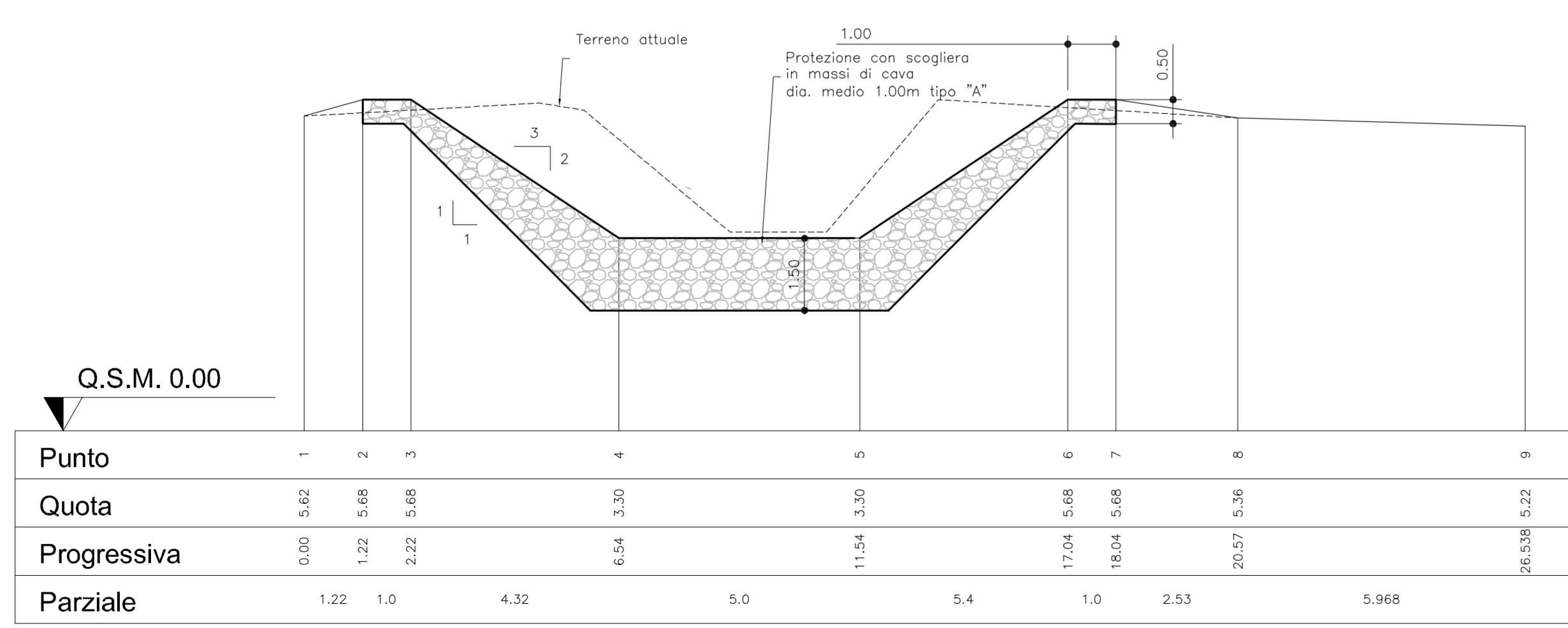
SEZIONE A-A
