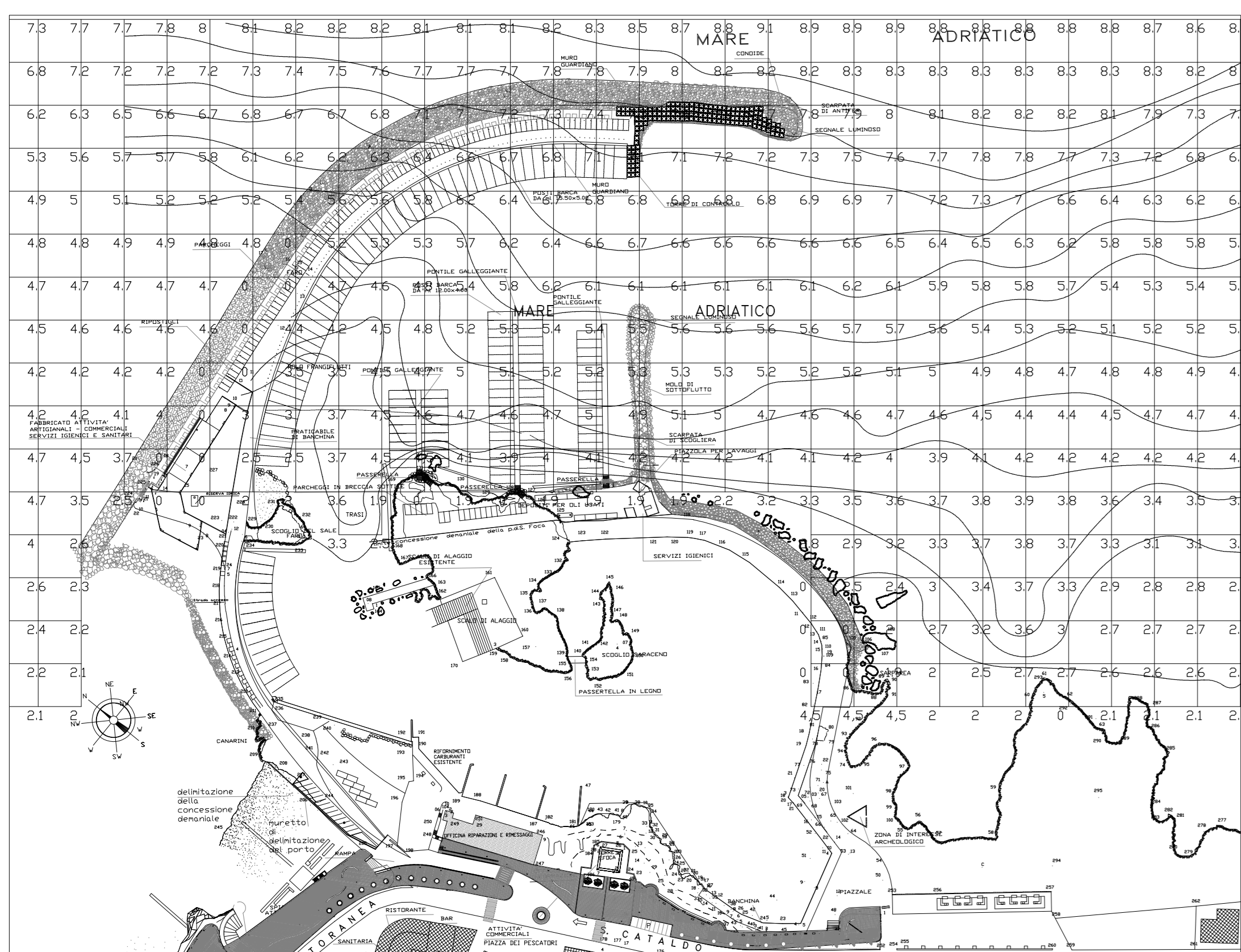
RILIEVO PLANIMETRICO E BATIMETRICO scala 1:2000
