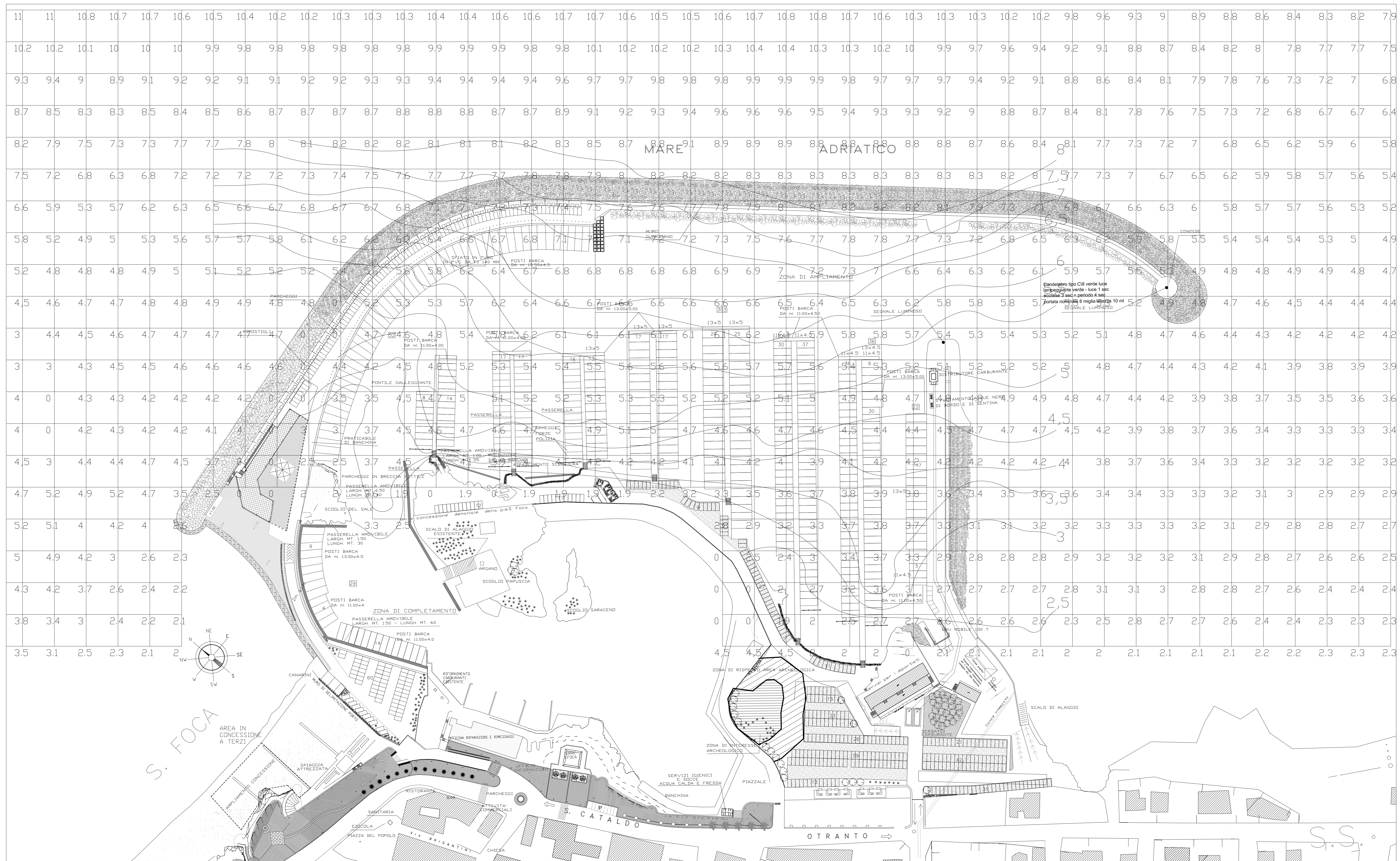
PLANIMETRIA DI PROGETTO scala 1:1000
