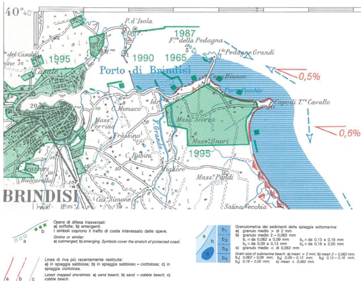
Figura 0-2. Estratto dell'Atlante delle Coste Italiane edito dal CNR
