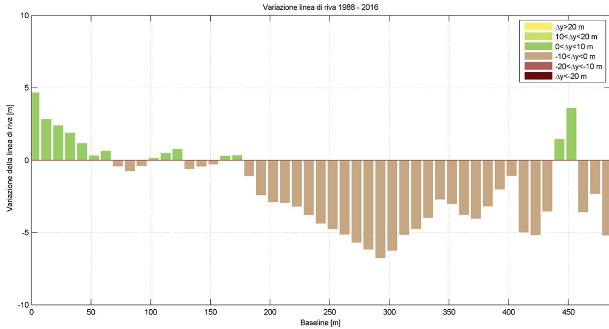
Figura 0-11. Variazione della linea di riva avvenuta tra il 1988 e il 2016.
