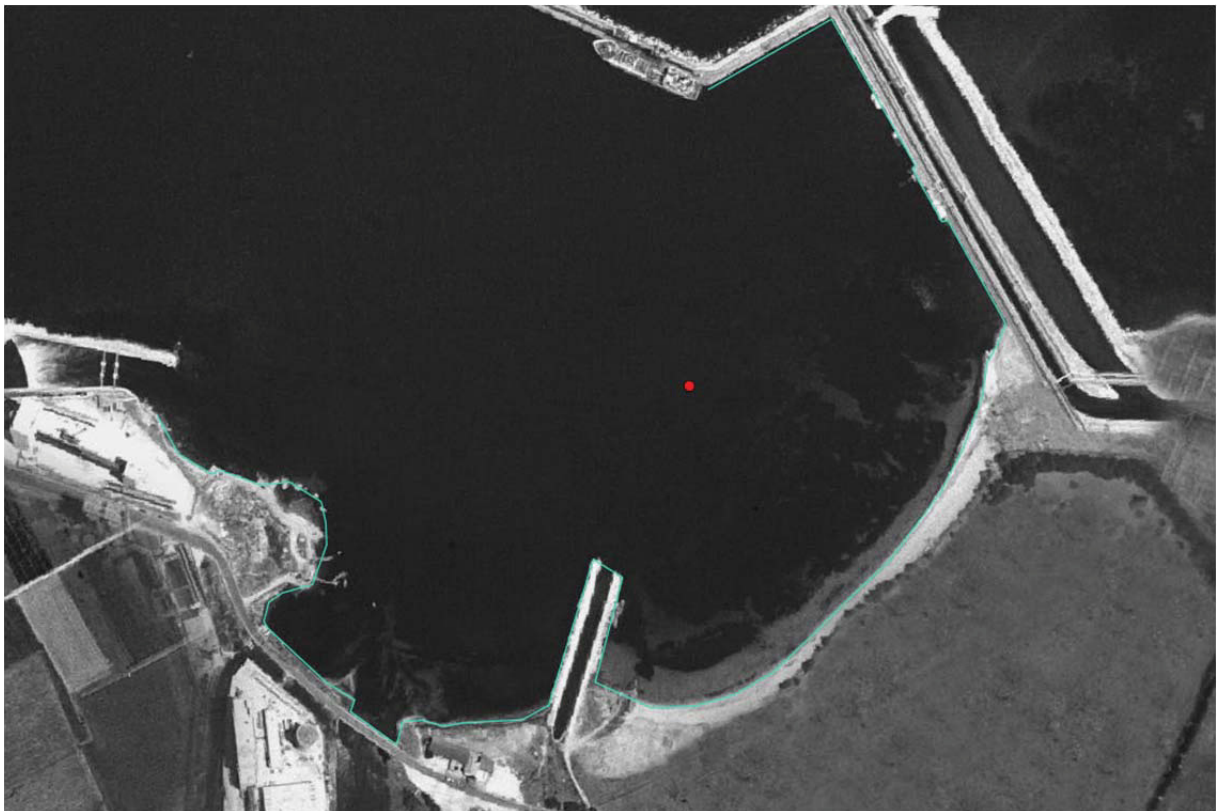
Figura 0-4. Evoluzione del litorale - Ortofoto 1994 (fonte: Portale Cartografico Nazionale).
