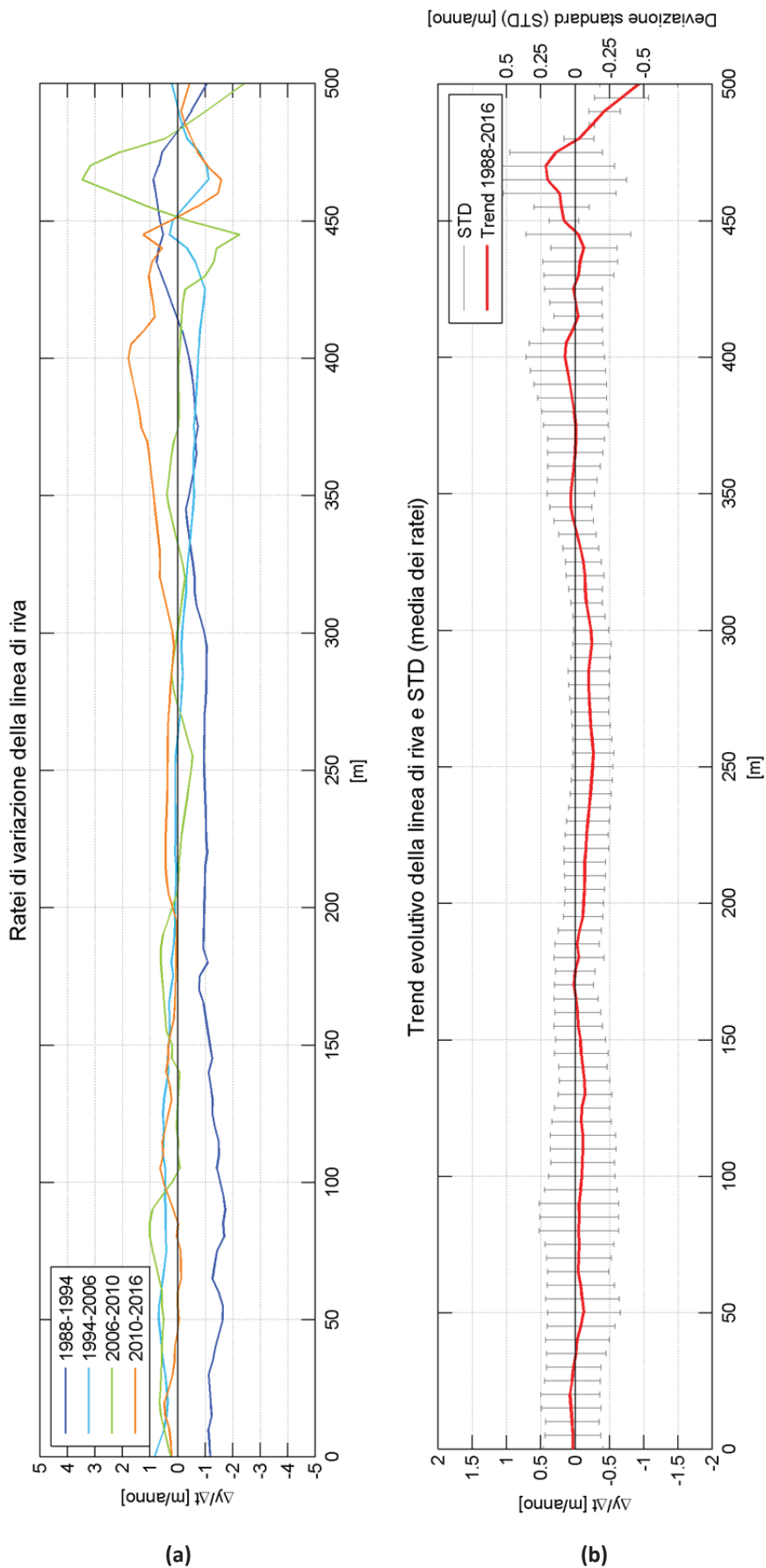
Figura 0-10 (a) Ratei di variazione calcolati tra i diversi intervalli temporali
