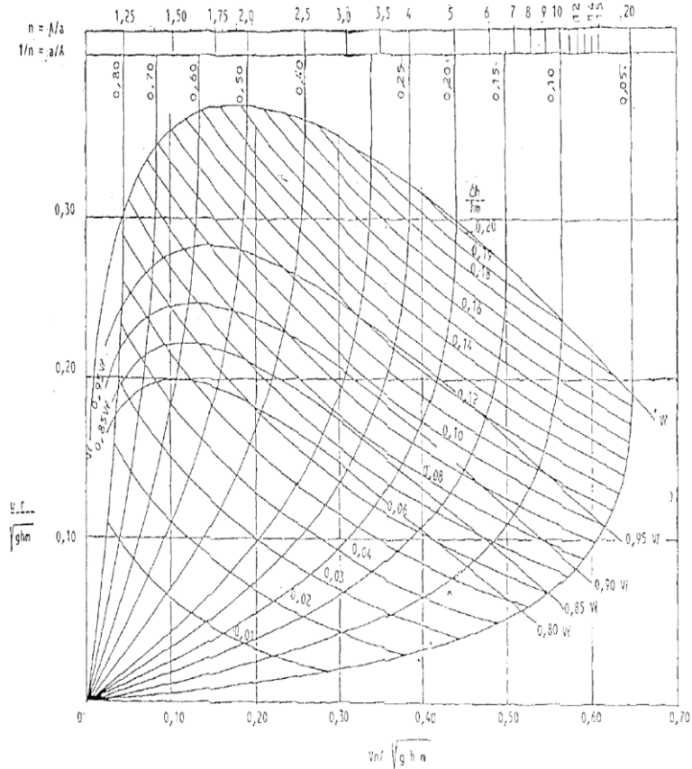
Diagramma di Schijf (modificato con coeff. di sicurezza 1,3) valori del rapporto tra la velocità limite e la velocità critica Vn / \sqrt{g h n} in funzione dell'indice di navigabilità n = A/a Valori della velocità della corrente di ritorno u_r e dell'abbassamento del piano d'acqua \delta h in funzione della velocità della nave Vn e dell'indice di navigabilità.
