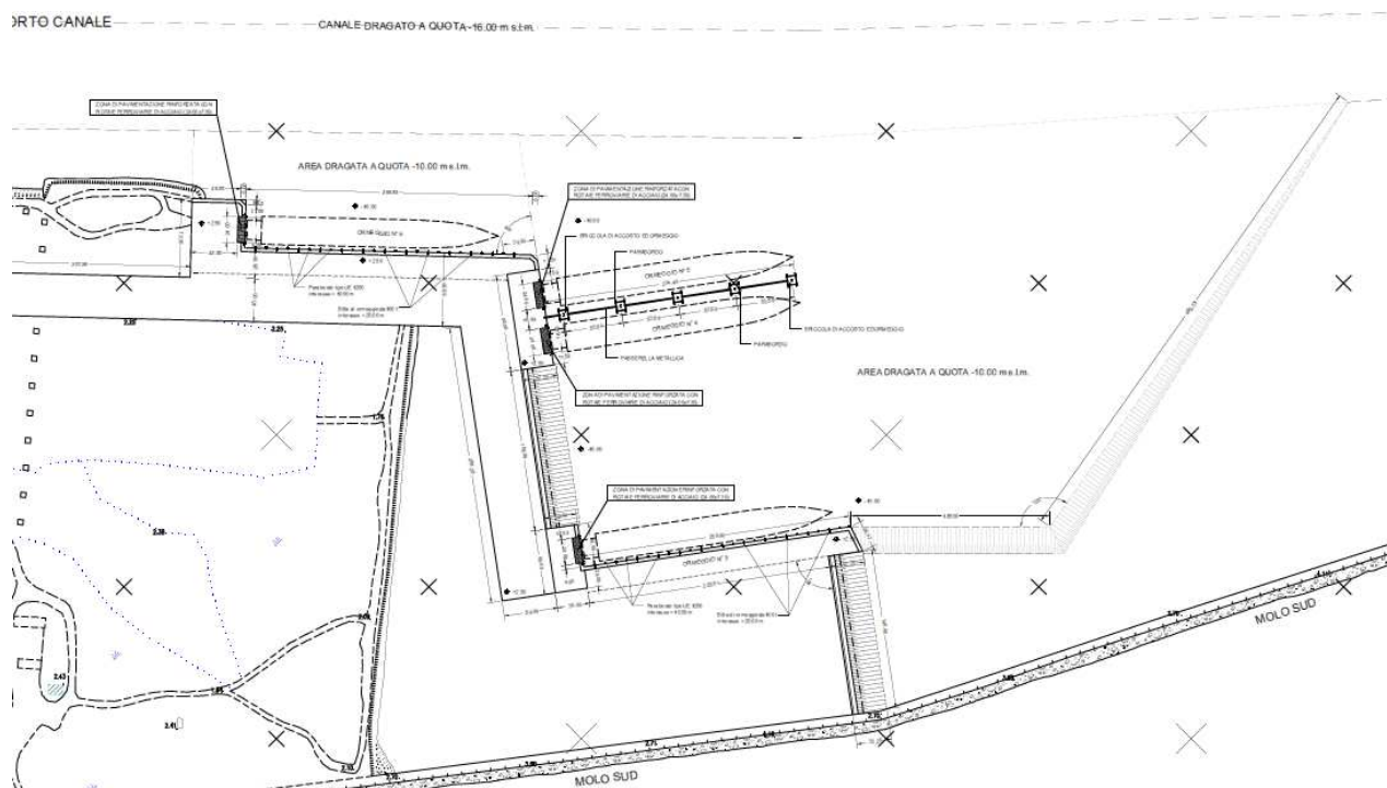
Figura 57 – Layout progettuale del I lotto funzionale del Terminal Ro Ro (Fonte: S.I.A. – Porto Canale di Cagliari – Terminal Ro-Ro – I° lotto funzionale VDP s.r.l. - Autorità Portuale).
