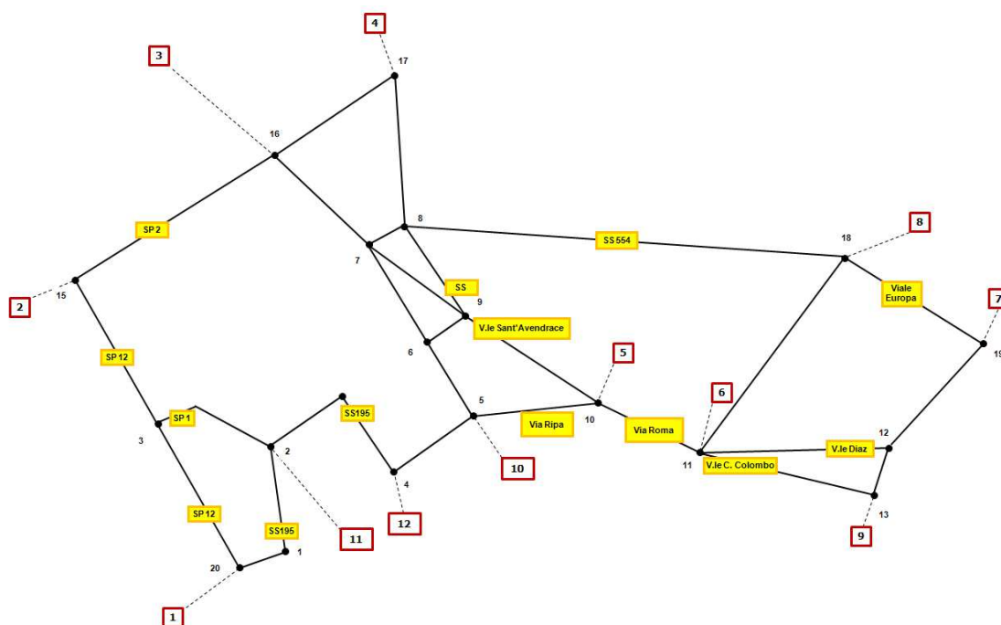
Figura 61 – Stralcio della rete viaria principale potenzialmente interessata dal transito dei mezzi connessi alla attività del Terminal Ro-Ro (Fonte: S.I.A. – Porto Canale di Cagliari – Terminal Ro-Ro – I° lotto funzionale VDP s.r.l. - Autorità Portuale).
