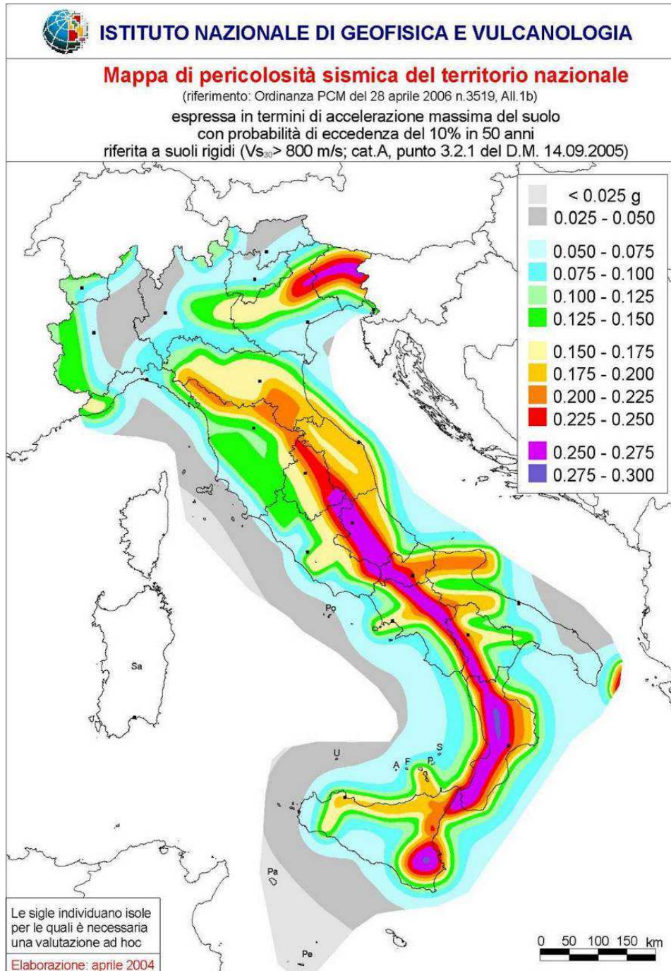
Figura 31 - Mapa della pericolosità sismica per il territorio nazionale.
