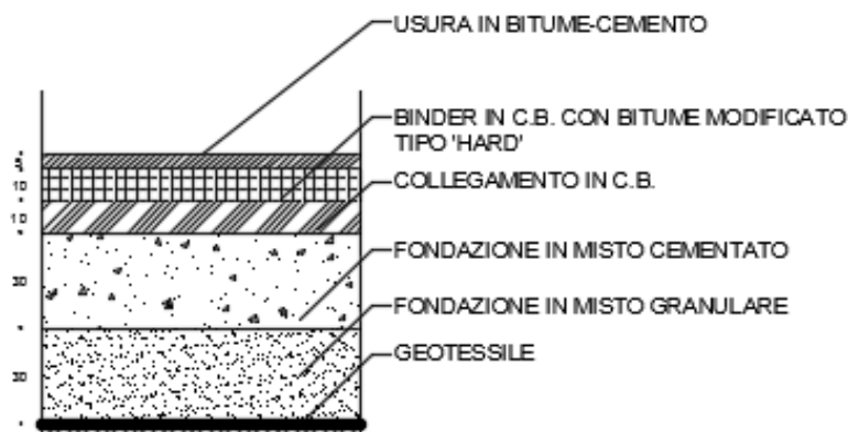
Figura 3.k: Pacchetto di Pavimentazione Viabilità e Aree di Passaggio / Sosta Automezzi
