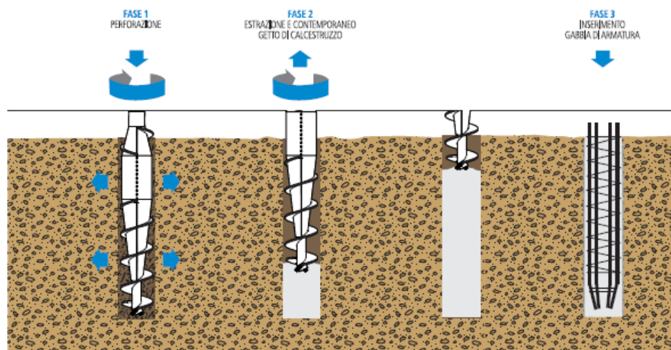
Figura 3.b: Pali Rotopressati a Costipamento Laterale
