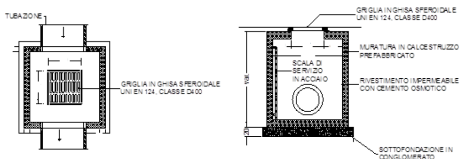
Figura 3.m: Dettaglio Tipologico Pozzetto
