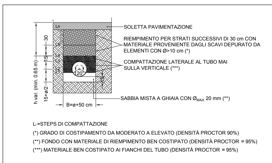
Figura 3.n: Dettaglio Posa Tubazioni PEAD
