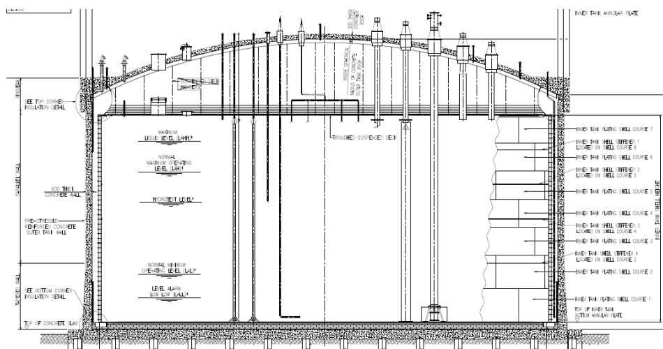
Figura 3.d: Serbatoio di Stoccaggio (Sezione)
