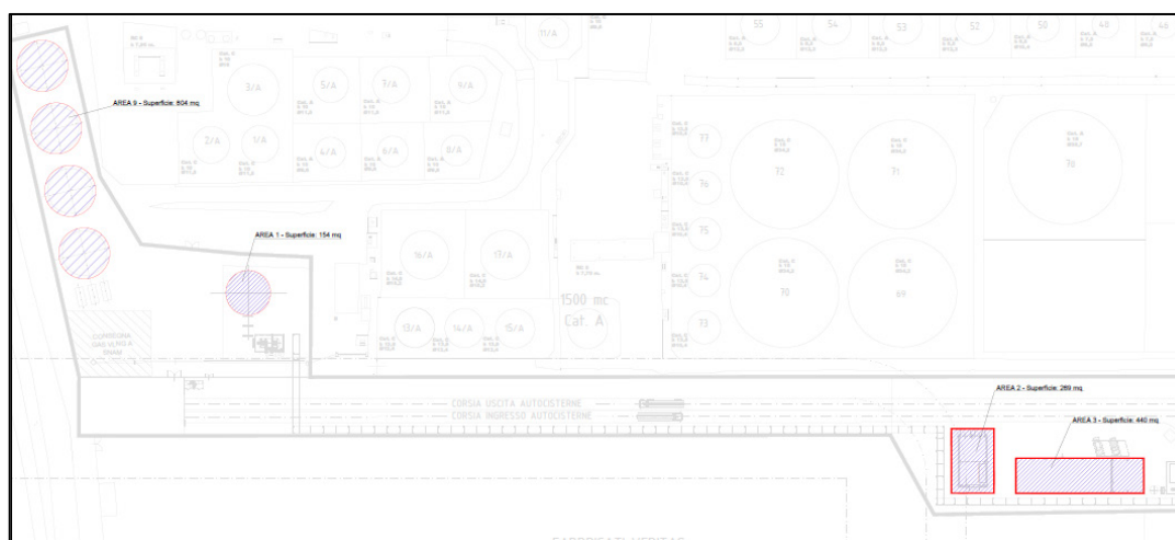
Figura 3.h: Planimetria delle Aree di Scavo a Sezione Obbligatoria per l'Area Sud dell'Impianto
