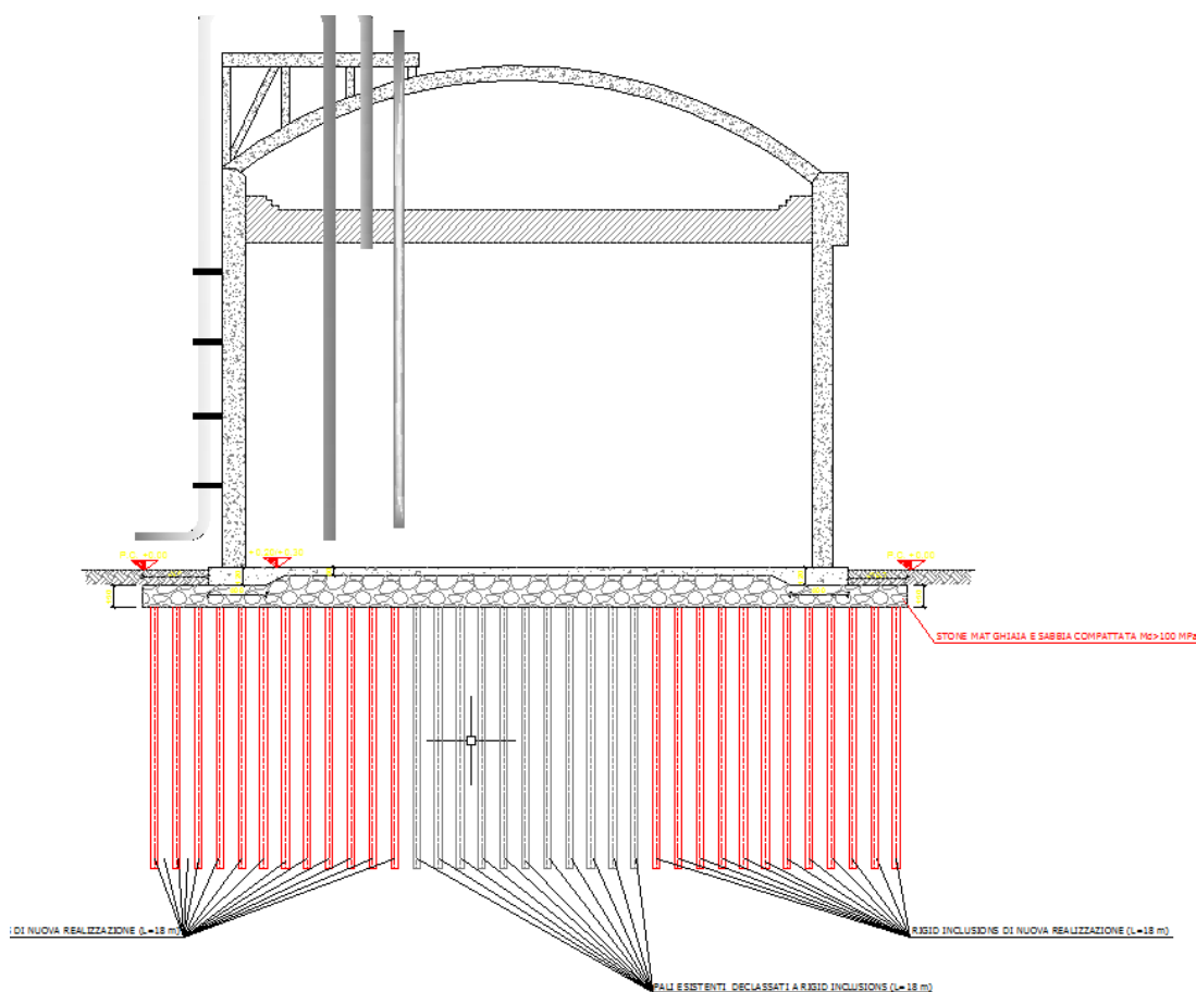
Figura 3.p: Sezione Fondazioni Serbatoio
