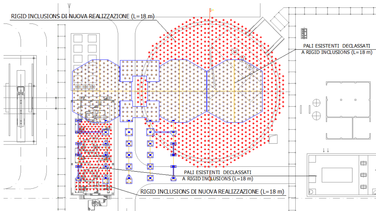
Figura 3.o: Pianta Fondazioni Serbatoio e Compressori
