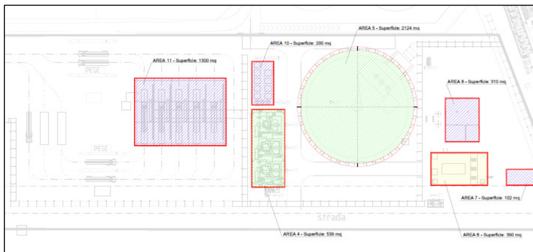
Figura 3.g: Planimetria delle Aree di Scavo a Sezione Obbligatoria per l'Area Nord dell'Impianto
