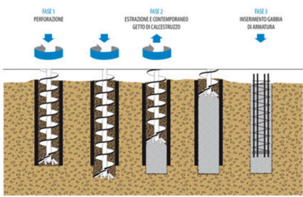
Figura 3.a: Pali a Elica Rivestiti con Camicia
