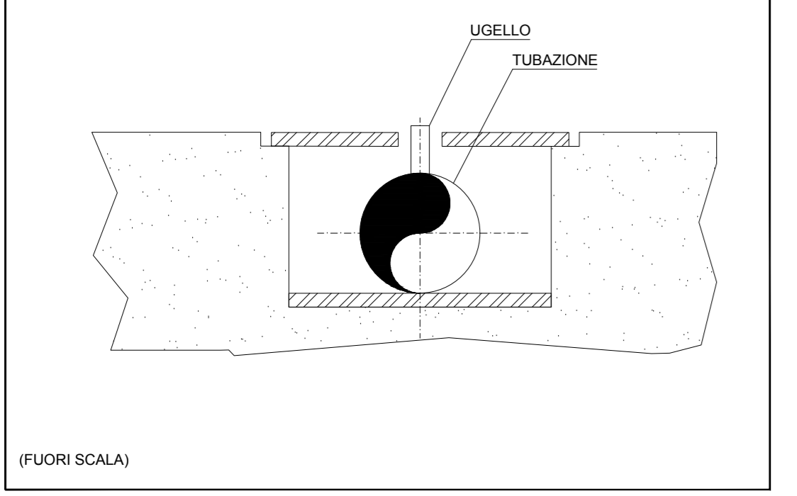
TIPICO SEZIONE TRASVERSALE BARRIERA AD ACQUA
