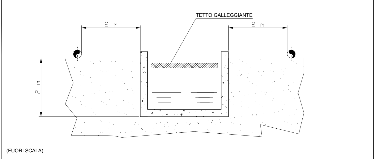
DETTAGLIO POSIZIONE BARRIERE AD ACQUA ATTORNO AI POZZETTI DI RACCOLTA
