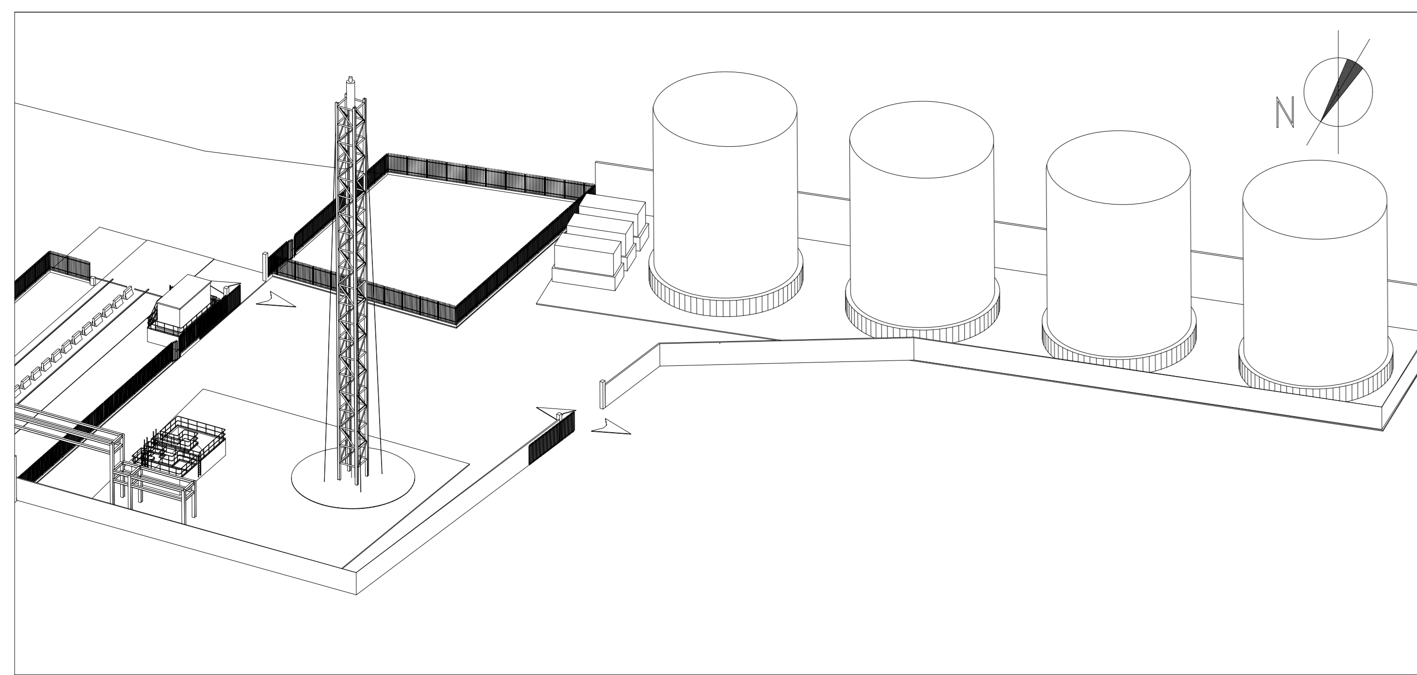
VISTA ASSONOMETRICA ZONA ANTINCENDIO E TORCIA
