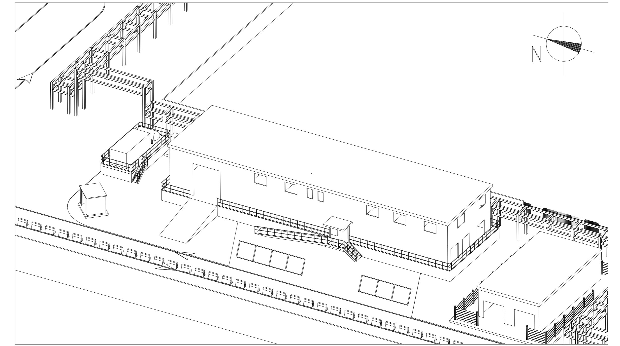
VISTA ASSONOMETRICA ZONA SALA CONTROLLO-UFFICI EDIFICIO ELETTRICO DIESEL D'EMERGENZA
