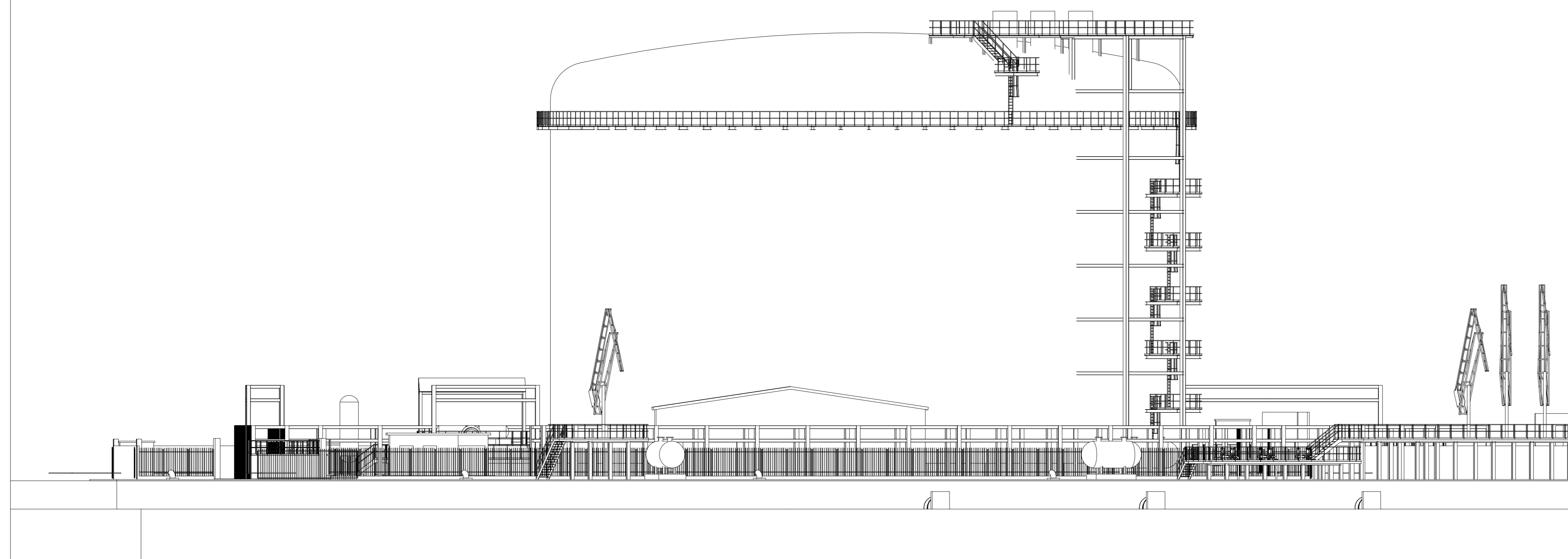
PROSPETTO NORD ZONA BANCHINA, STOCCAGGIO E GESTIONE B.O.G.
