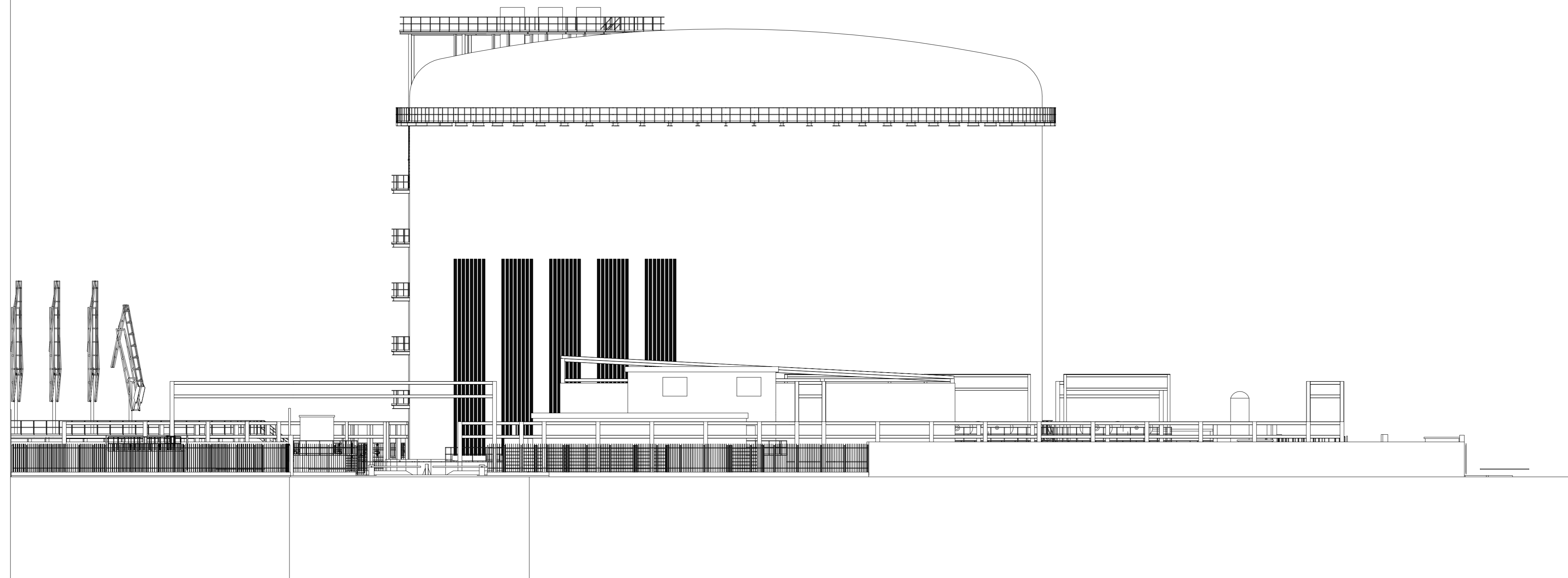
PROSPETTO NORD ZONA BANCHINA, STOCCAGGIO E GESTIONE B.O.G.
