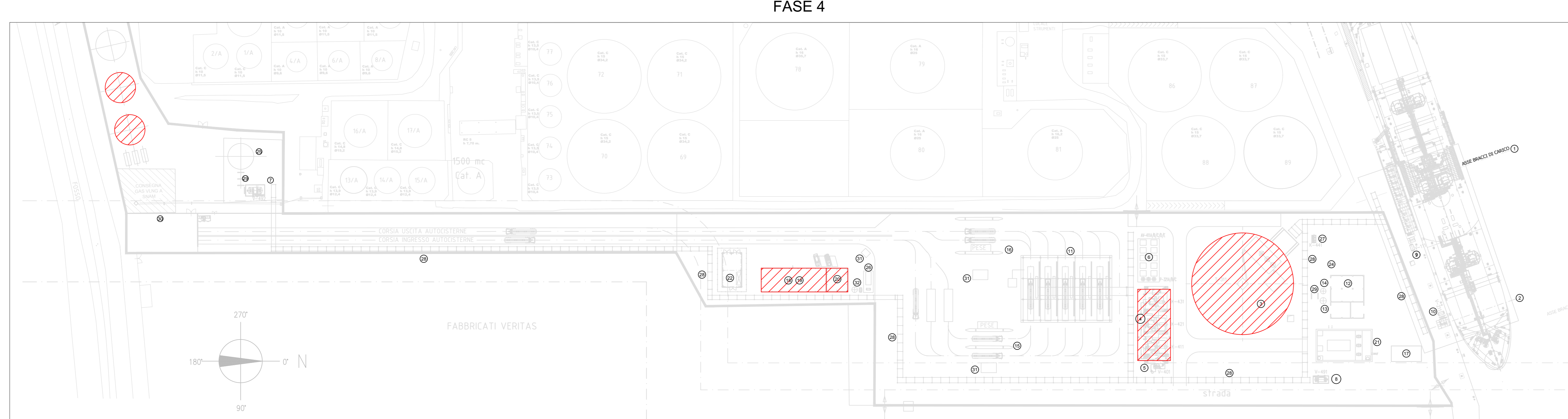
FASE 4: - FONDAZIONI SERBATOIO GNL - MAGAZZINO - FONDAZIONE COMPRESSORI - INSTALLAZIONE N° 2 SERBATOI ANTINCENDIO/DI RIUSO - SALA CONTROLLO - UFFICI - EDIFICIO ELETTRICO
