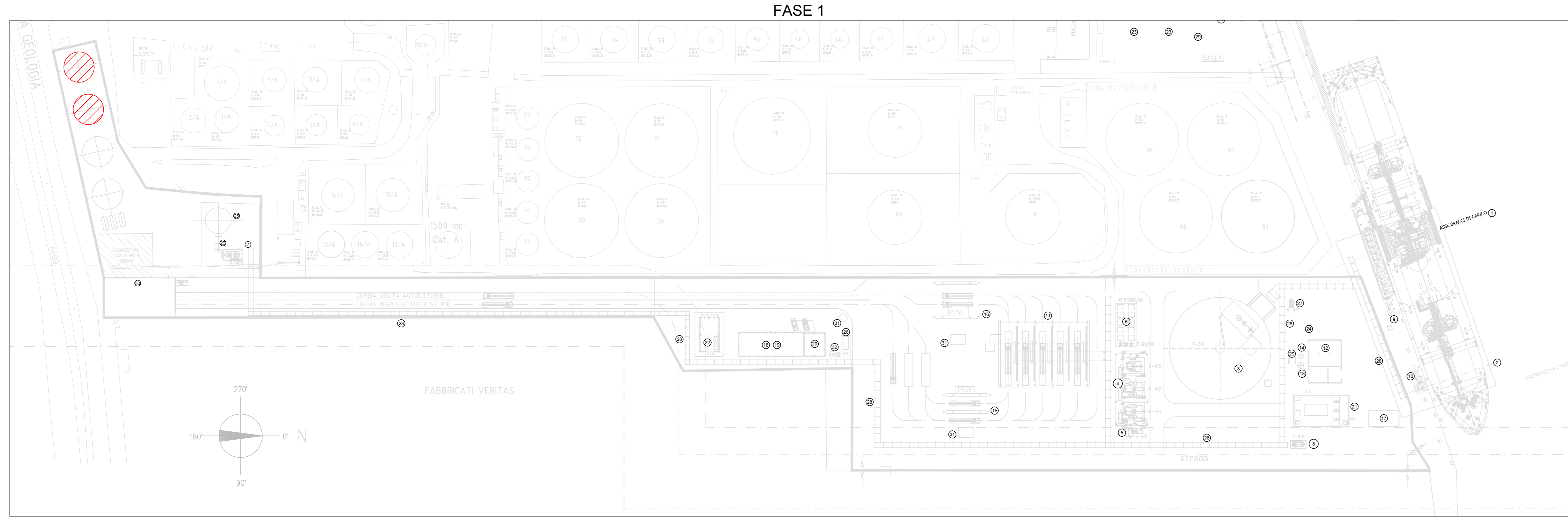
FASE 1: - INSTALLAZIONE n° 2 SERBATOI ANTINCENDIO/DI RIUSO
