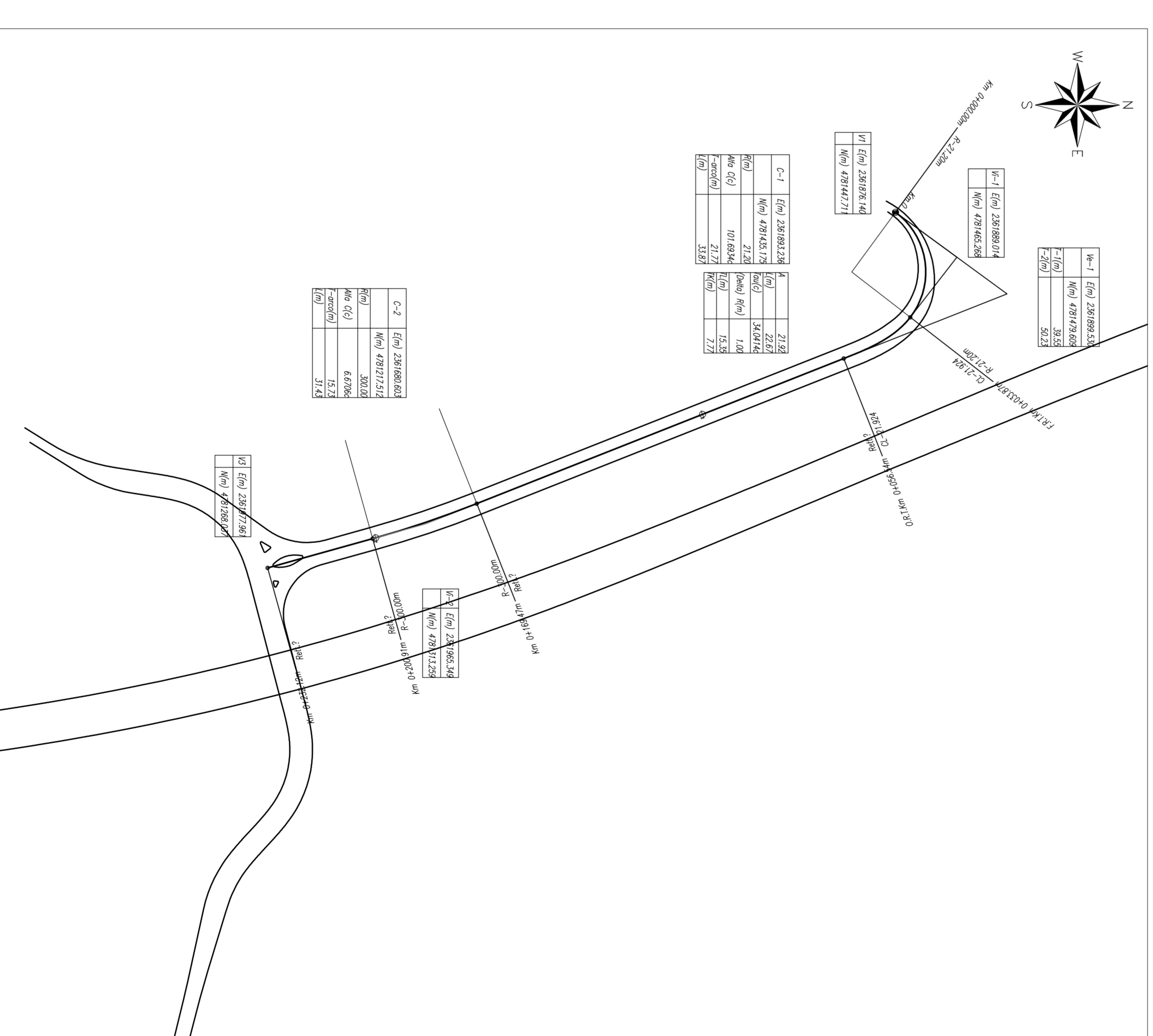
Planimetria di tracciamento viabilità di collegamento strada podereale - strada di via Berta - Scala - 1:1000
