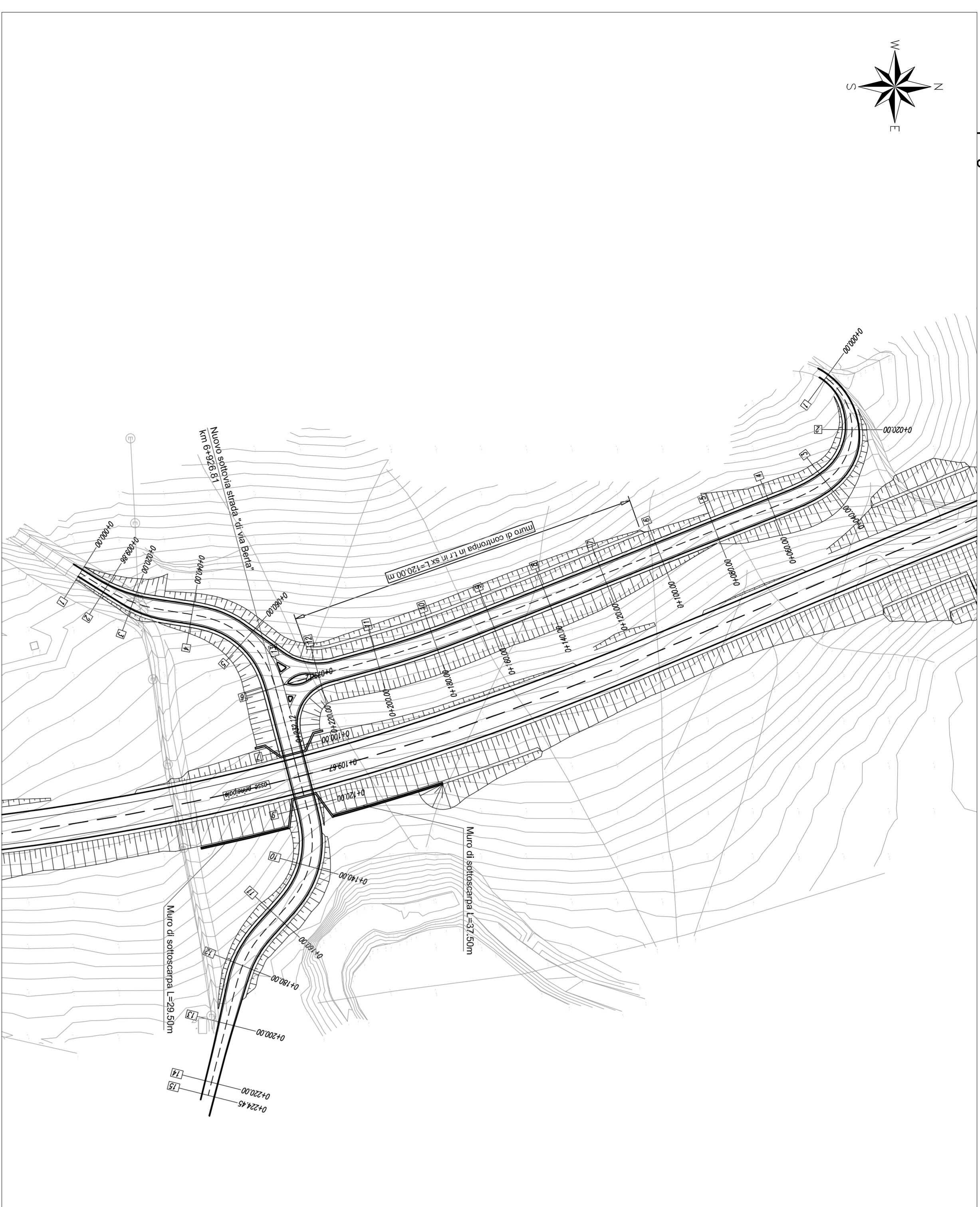
Planimetria di progetto - Scala - 1:1000
