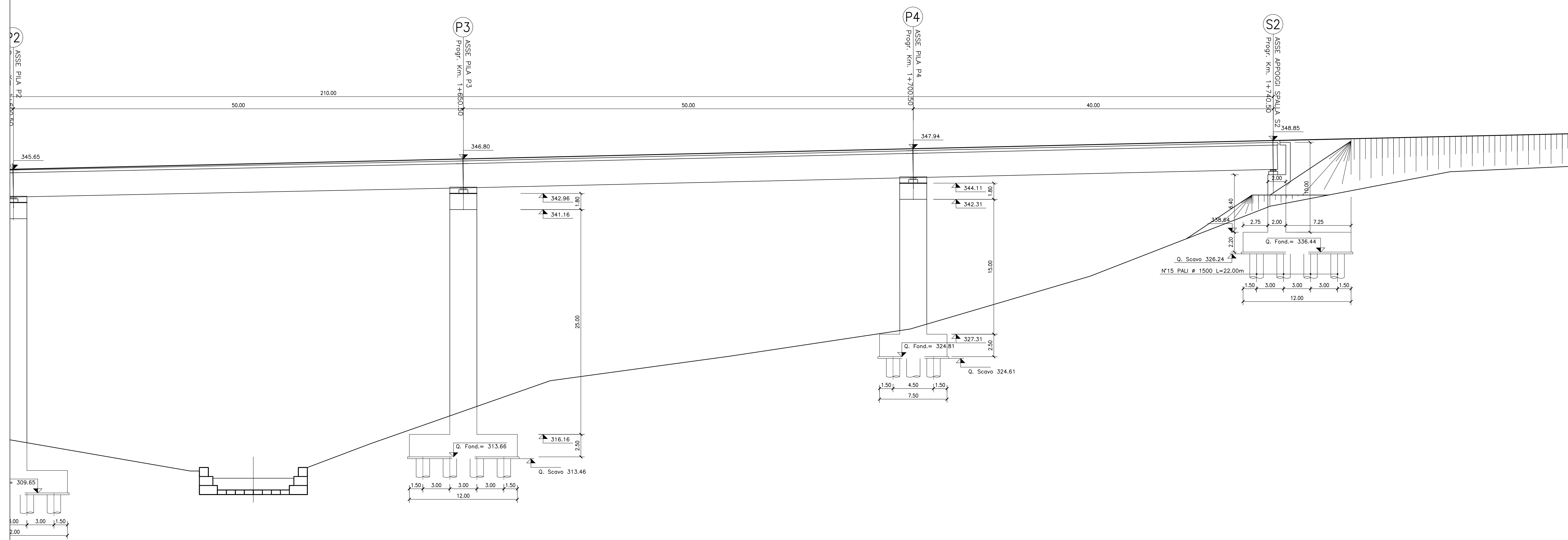
PROSPETTO LONGITUDINALE Scala 1:200
