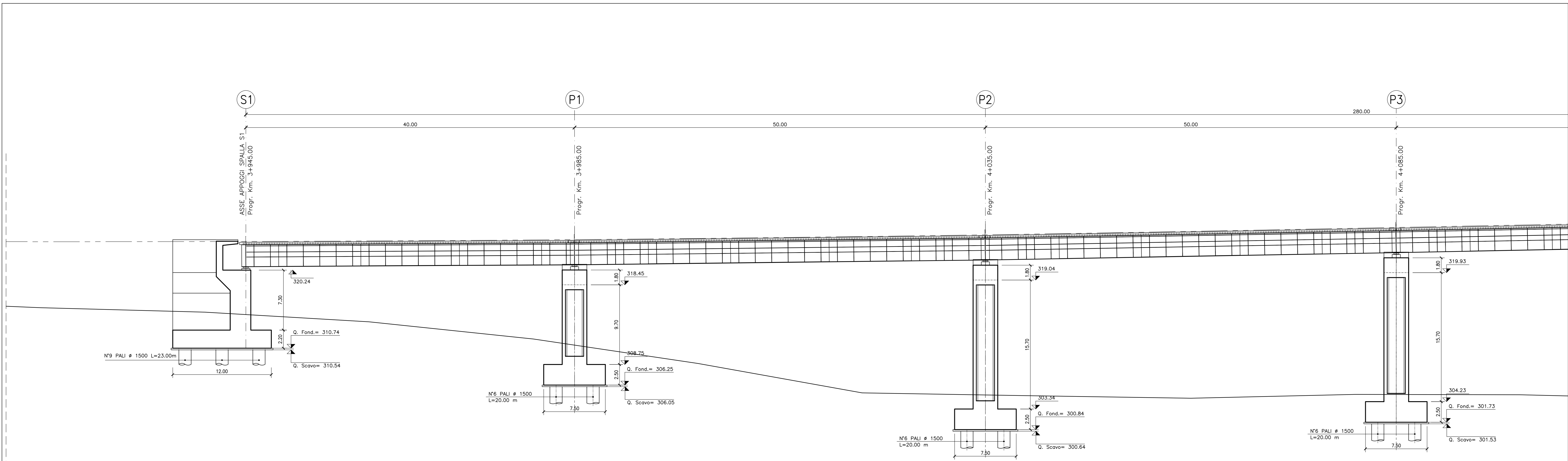
PROFILO LONGITUDINALE Scala 1:200
