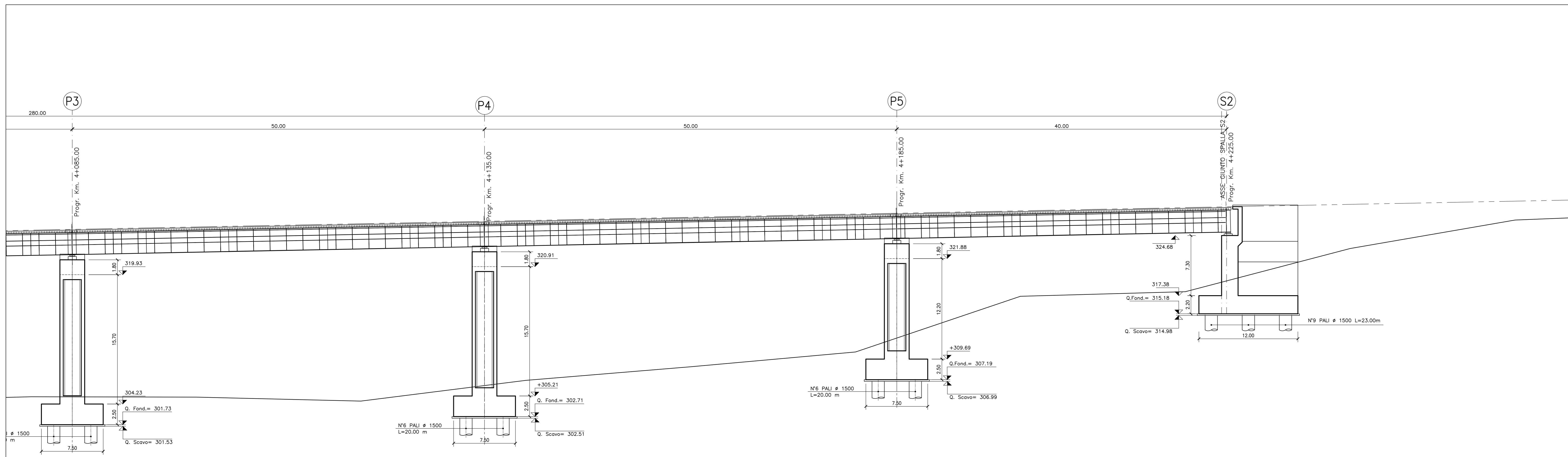
SEZIONE LONGITUDINALE IN ASSE VIADOTTO Scala 1:200
