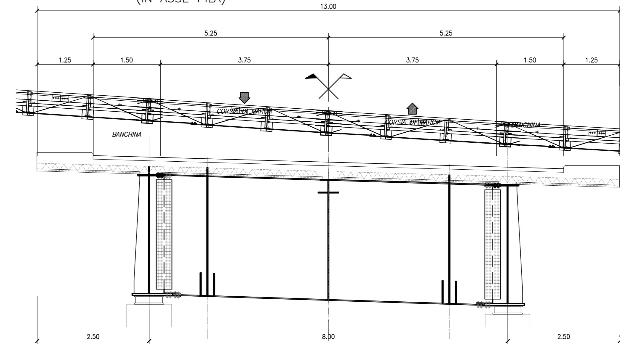
IMPALCATO - SEZIONE TRASVERSALE - Scala 1:50 (IN ASSE PILA)
