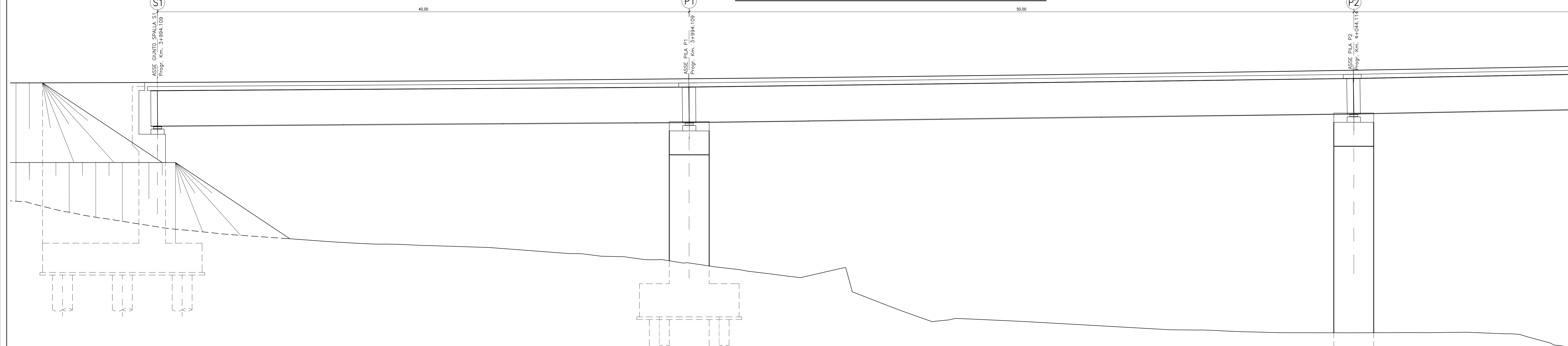
SEZIONE LONGITUDINALE IN ASSE IMPALCATO - Scala 1:100
