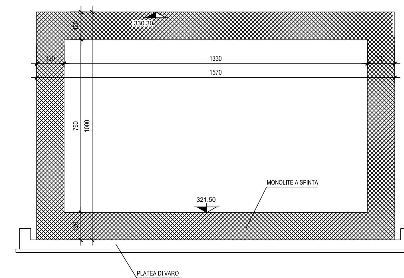
SEZIONE TRASVERSALE MONOLITE A SPINTA - SCALA 1: 100 -
