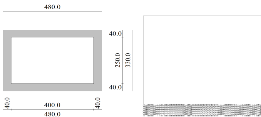
Modello Geometrico Geotecnico di Riferimento – 2/2
