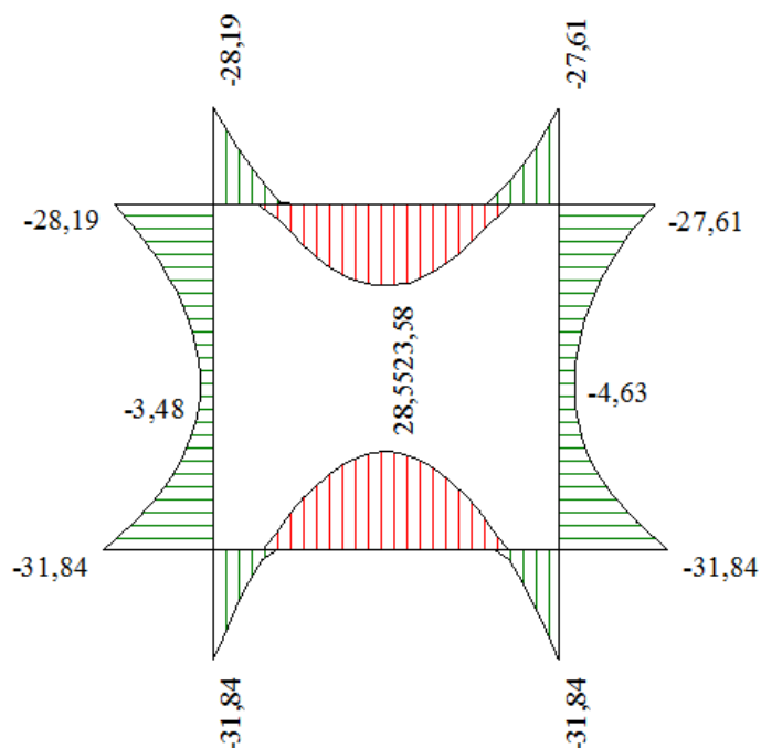
Inviluppo diagrammi del momento flettente – SLE
