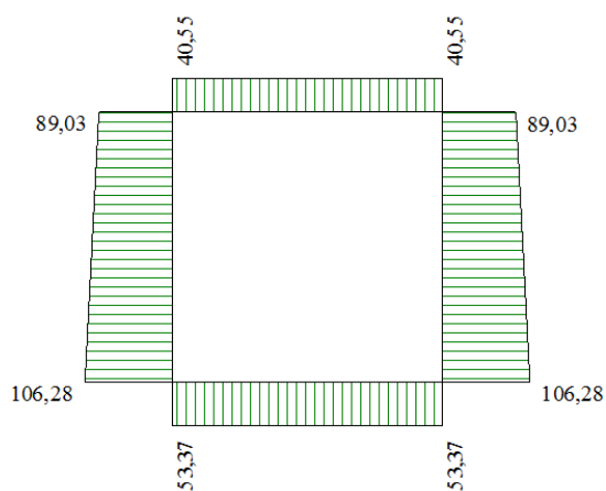
Inviluppo diagrammi dello sforzo normale – SLE
