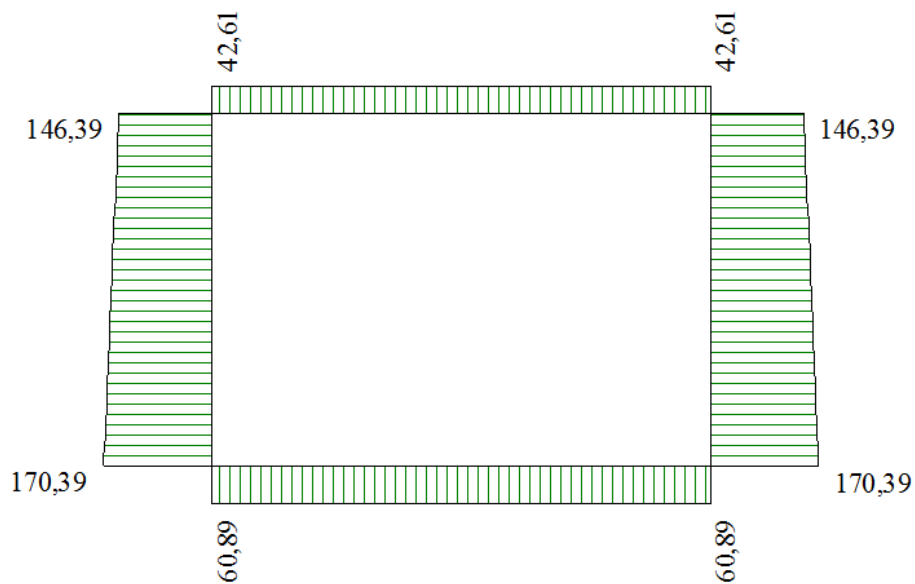
Inviluppo diagrammi dello sforzo normale – SLE
