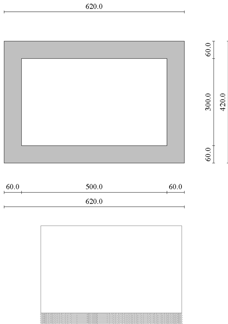
Modello Geometrico Geotecnico di Riferimento – 2/2
