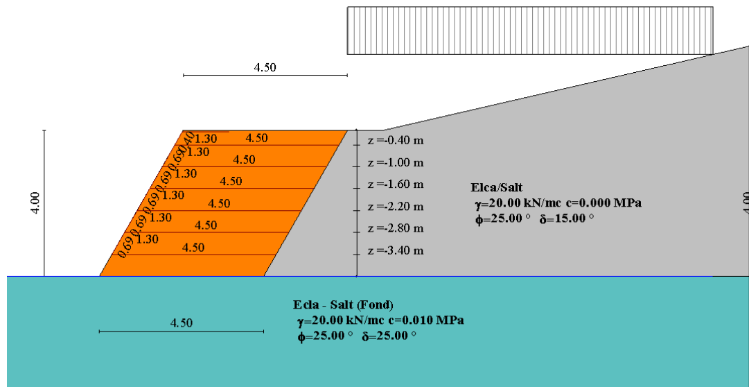
Modello Geometrico e Geotecnico
