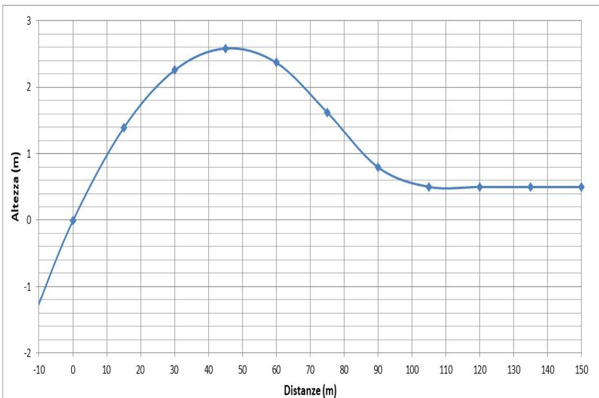
Figura 13 – Calcolo e grafico della curva di varo per angolo di uscita 8°, raggio 420 m. Altezza max. = 2.59 m
