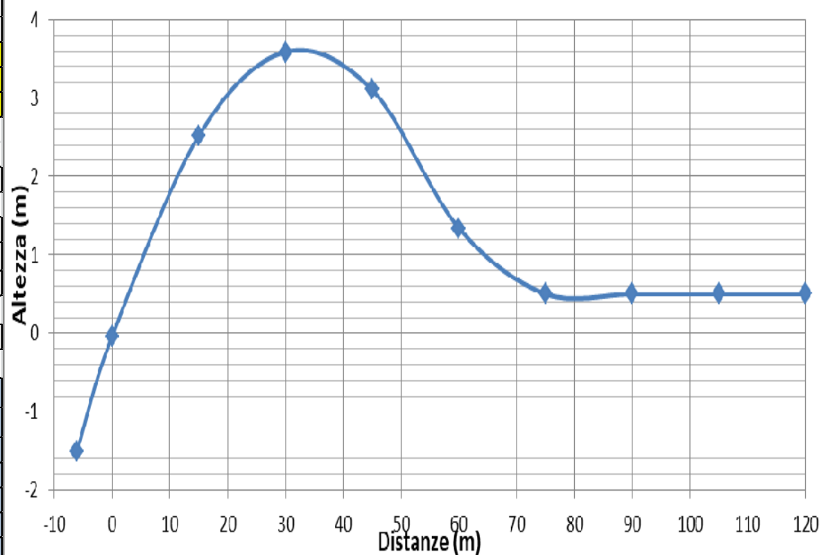
Figura 13 – Calcolo e grafico della curva di varo per angolo di uscita 15°, raggio 150 m. Altezza max. = 3.61 m
