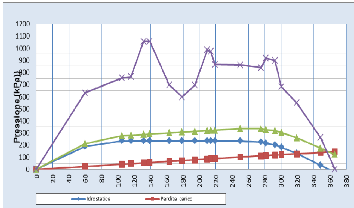
Figura 12 - Andamento della pressione operativa e della resistenza del terreno in funzione della distanza dall'entrata
