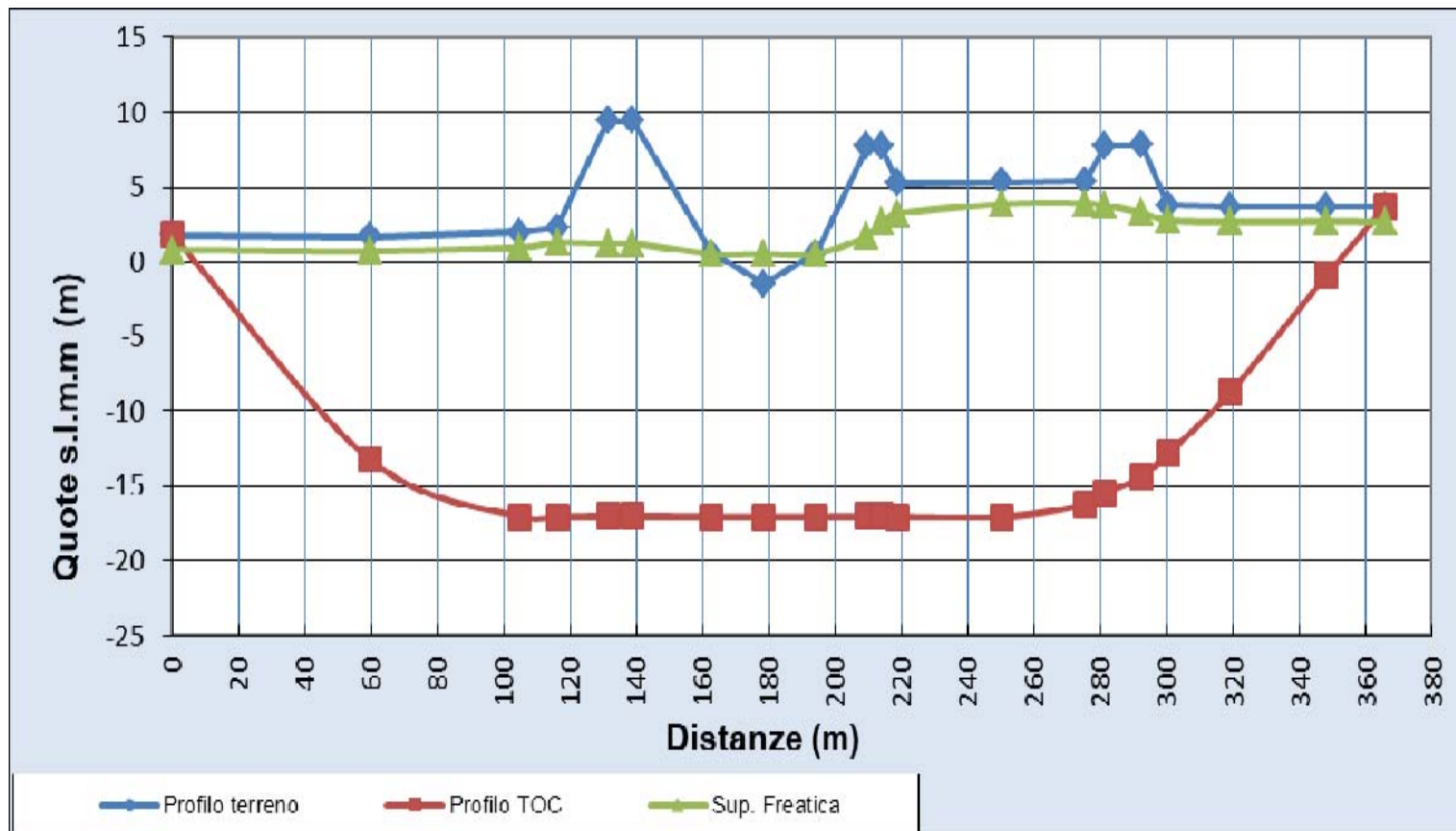
Figura 11 –Sezione schematica del terreno e della T.O.C. (entrata della trivellazione a sinistra)
