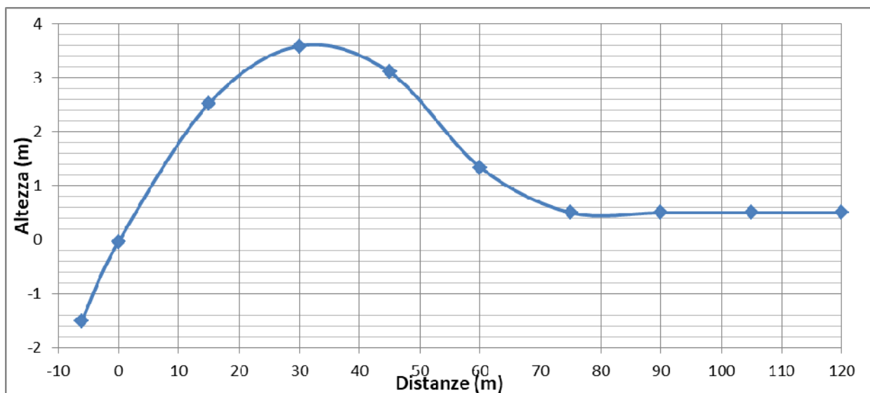
Figura 6 – Grafico della curva di varo nell'ipotesi di angolo di uscita di 15^\circ e raggio= 150 m
