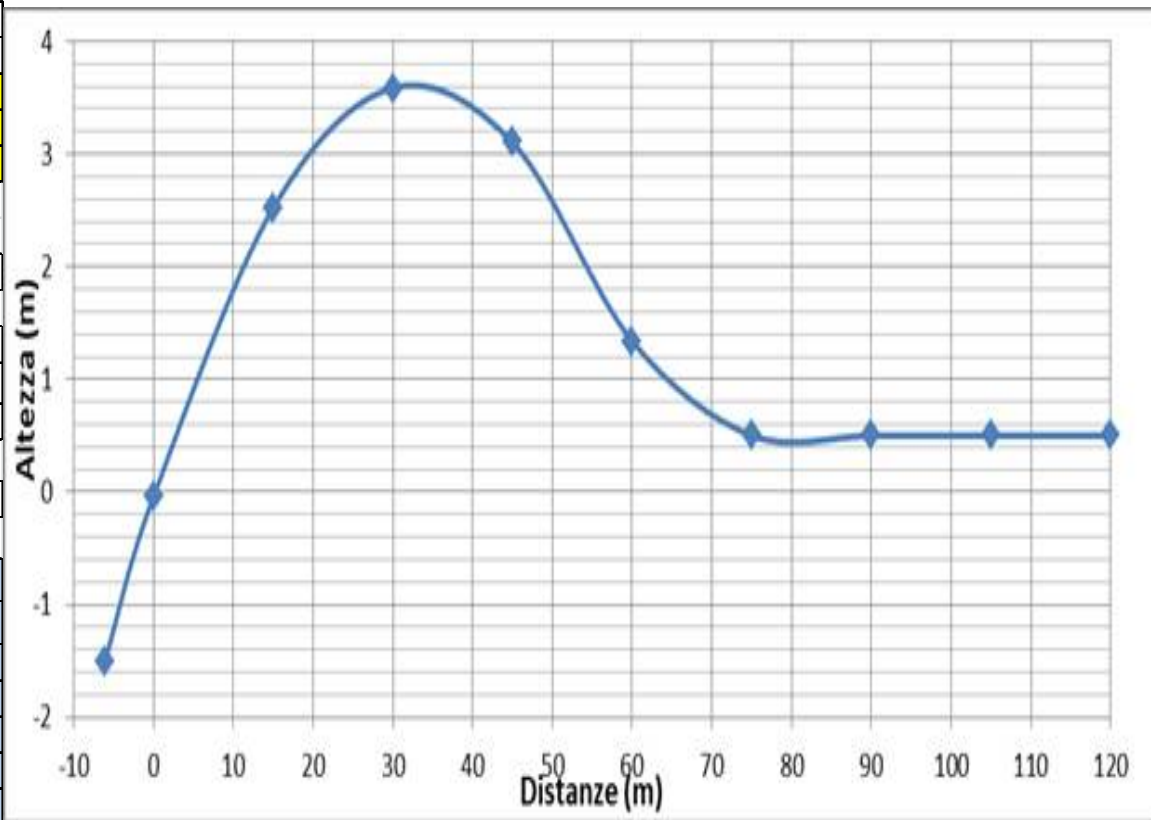
Figura 13 – Calcolo e grafico della curva di varo per angolo di uscita 15°, raggio 150 m. Altezza max. = 3.61 m
