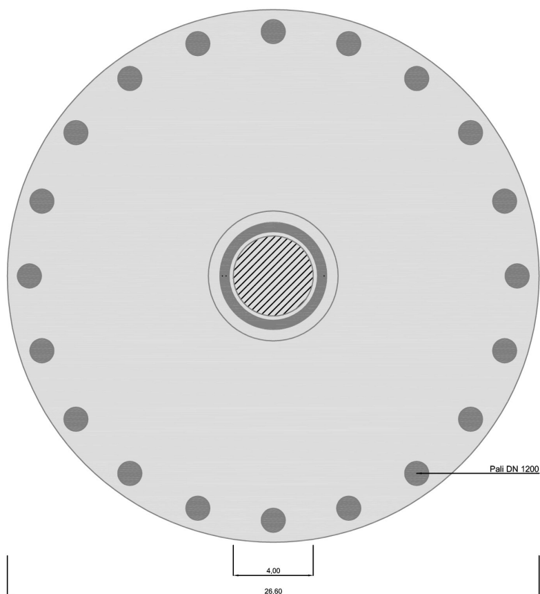
PIANTA FONDAZIONE TIPO Scala 1:100
