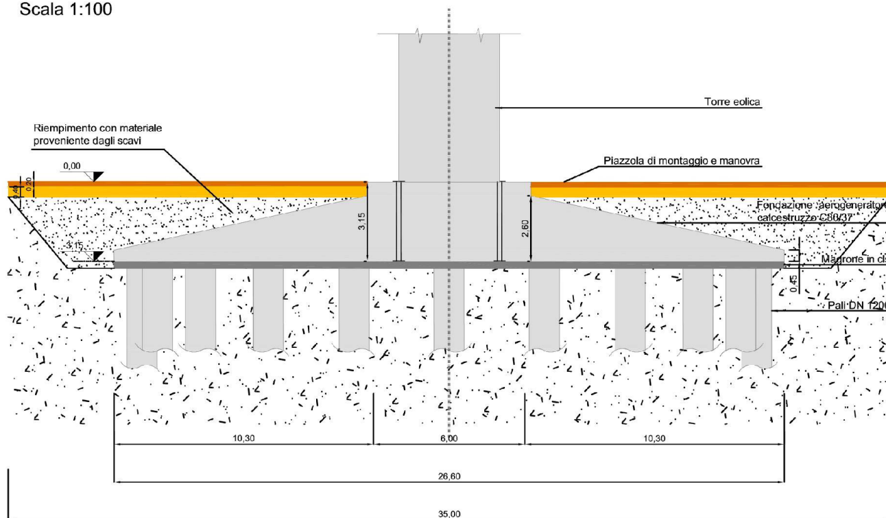
Fig. 1: Sezione fondazione tipo
