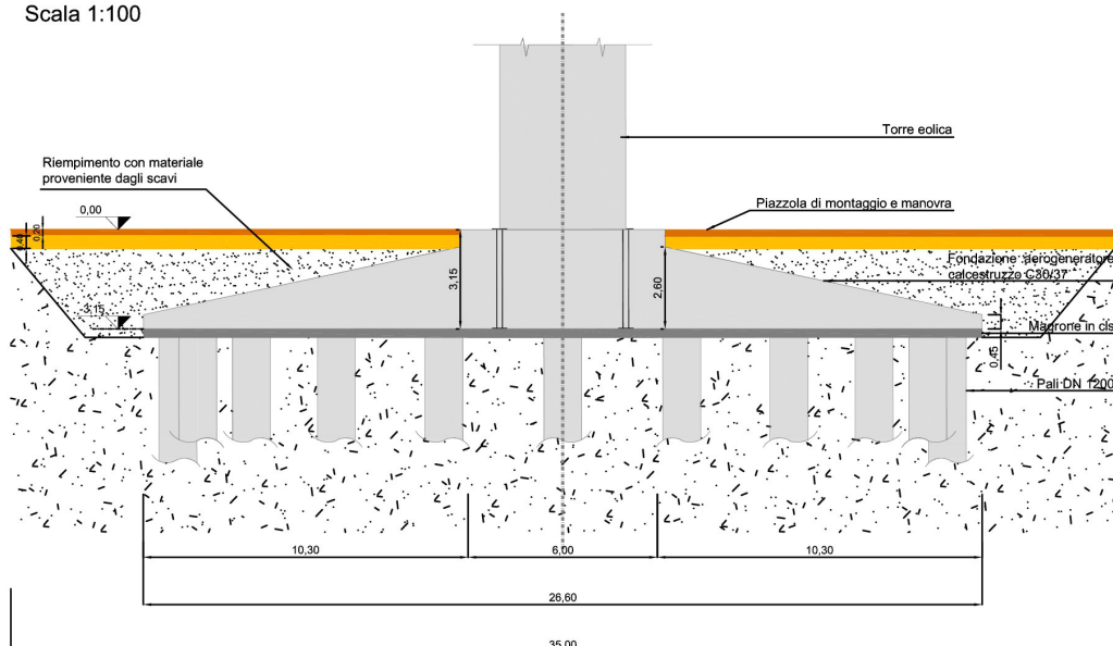
SEZIONE PIAZZOLA E FONDAZIONE TIPO Scala 1:100
