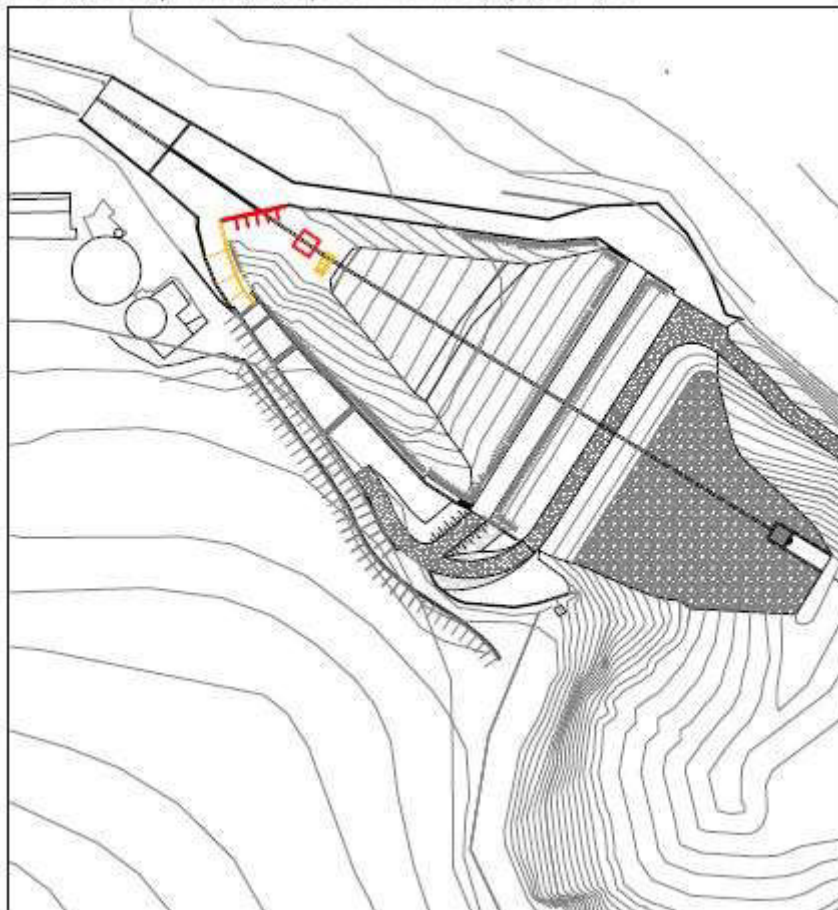
FASE 7: Interventi pozzetto di valle e parete monte vasca di dissipazione - 1:1000
