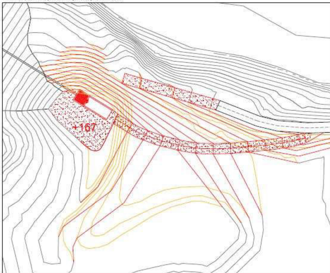
FASE 3: Interventi pozzetto opera di presa - 1:500
