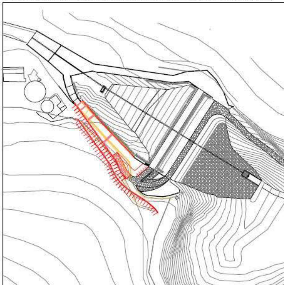
FASE 5/6: Interventi strada adiacente scollatore sinistro e scollatore da sezione 4 a sezione 10a - 1:1000
