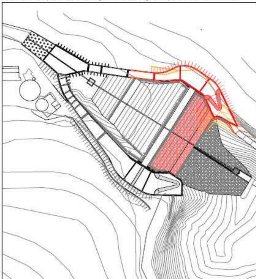
FASE 12/13; Completamento canale fugalore destro e scogliera su paramento di monte - 1:1000
