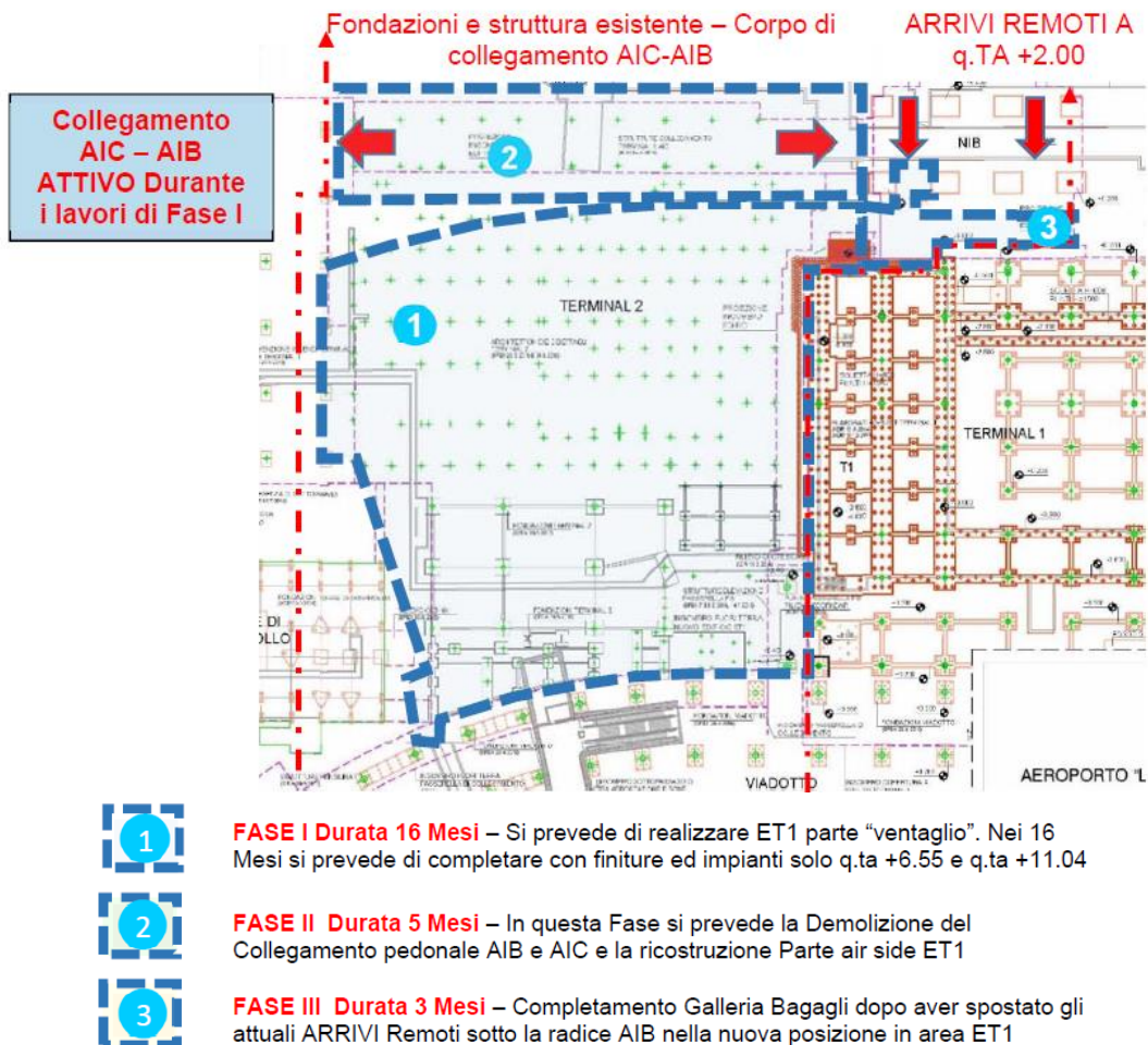
Figura 2-3 Pianta Fondazioni e Corpo di Collegamento esistente
