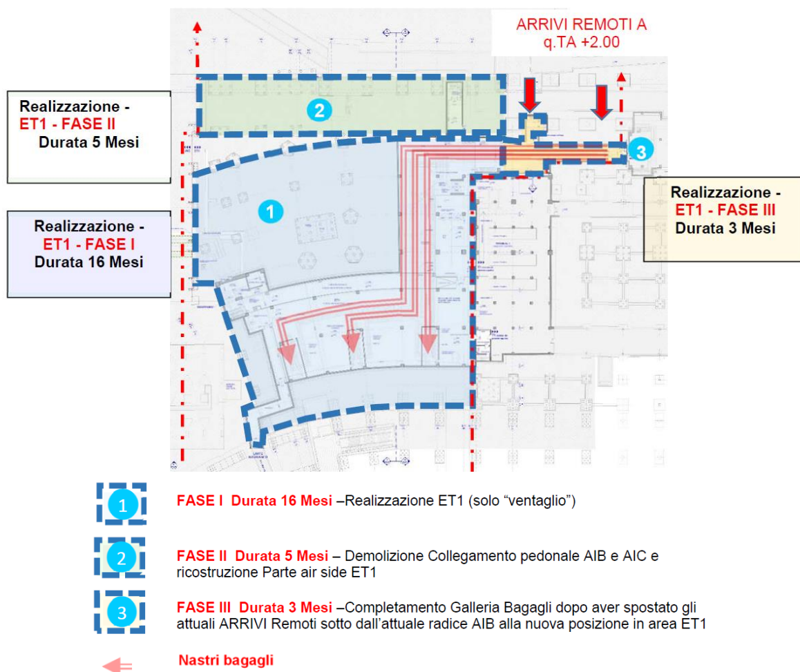
Figura 2-2 Piano Interrato e Galleria Bagagli
