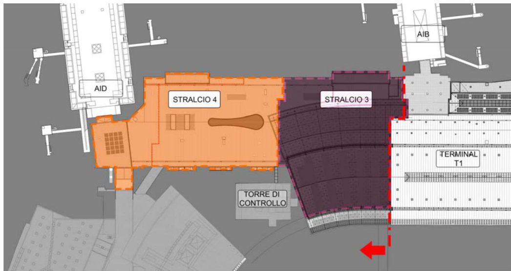
Figura 1-2 Lotto 2: aree funzionali di intervento stralcio 3 e 4
