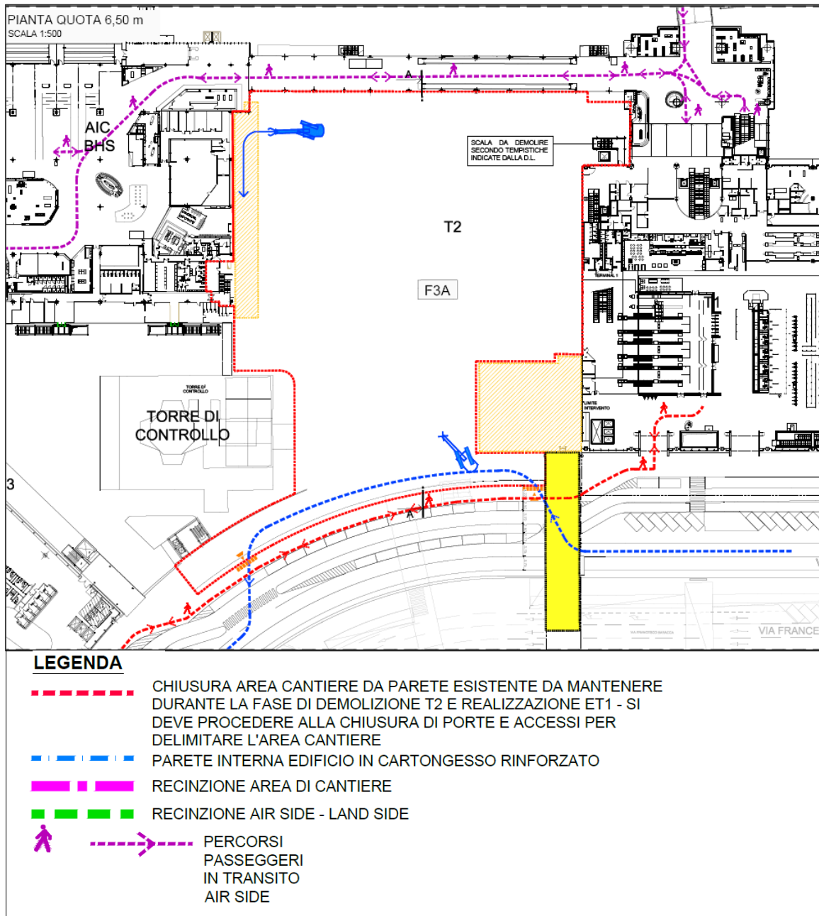
Figura 3-2 Stralcio tavola STR DEM 008
