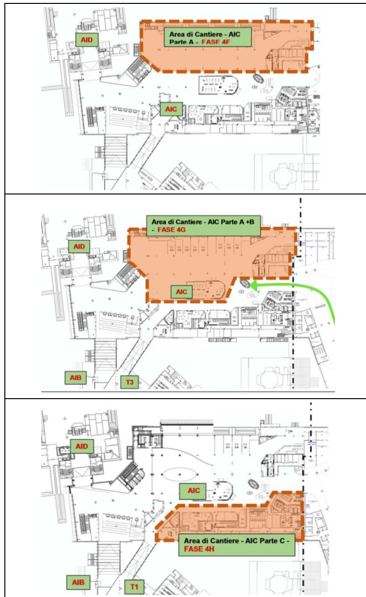
Figura 2-6 Piano q.ta +1.72 – Livello piazzali (Fase 4F, 4G, 4H)
