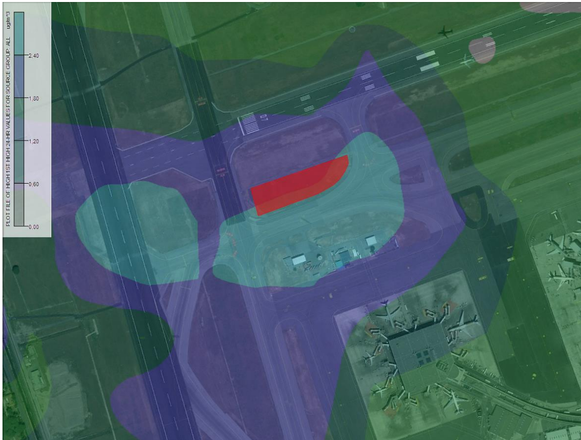
Figura 7-11 Massimi sulla maglia di calcolo media 24h PM 10 Fase 1
