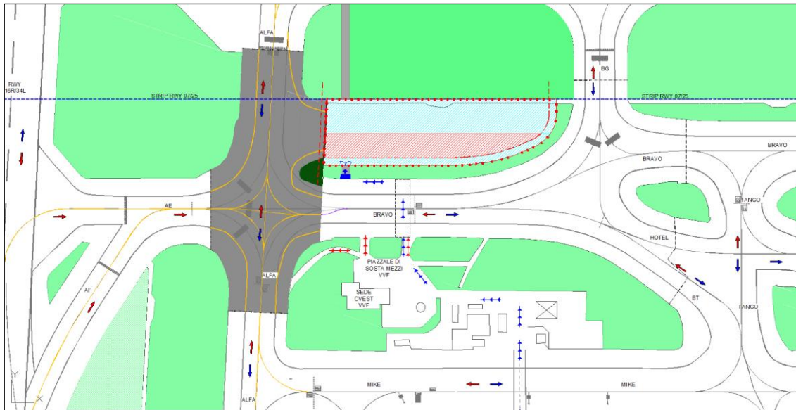
Figura 7-9 Area di cantiere
