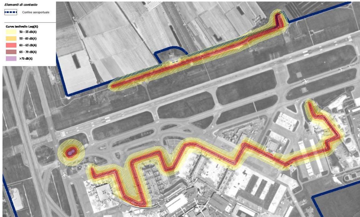
Figura 7-14 Curve di isolivello acustico indotte da sorgenti di cantiere e dal trasporto dei materiali, nel periodo diurno
