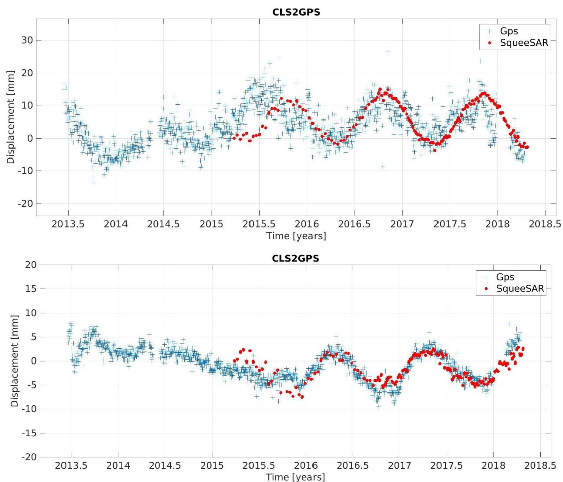
Figura 4: Confronto tra la serie storica della componente verticale (in alto) e la componente est-ovest (in basso) fornita dalla stazione GNSS e quella ottenuta dalla combinazione dei dati satellitari acquisiti in doppia geometria.
