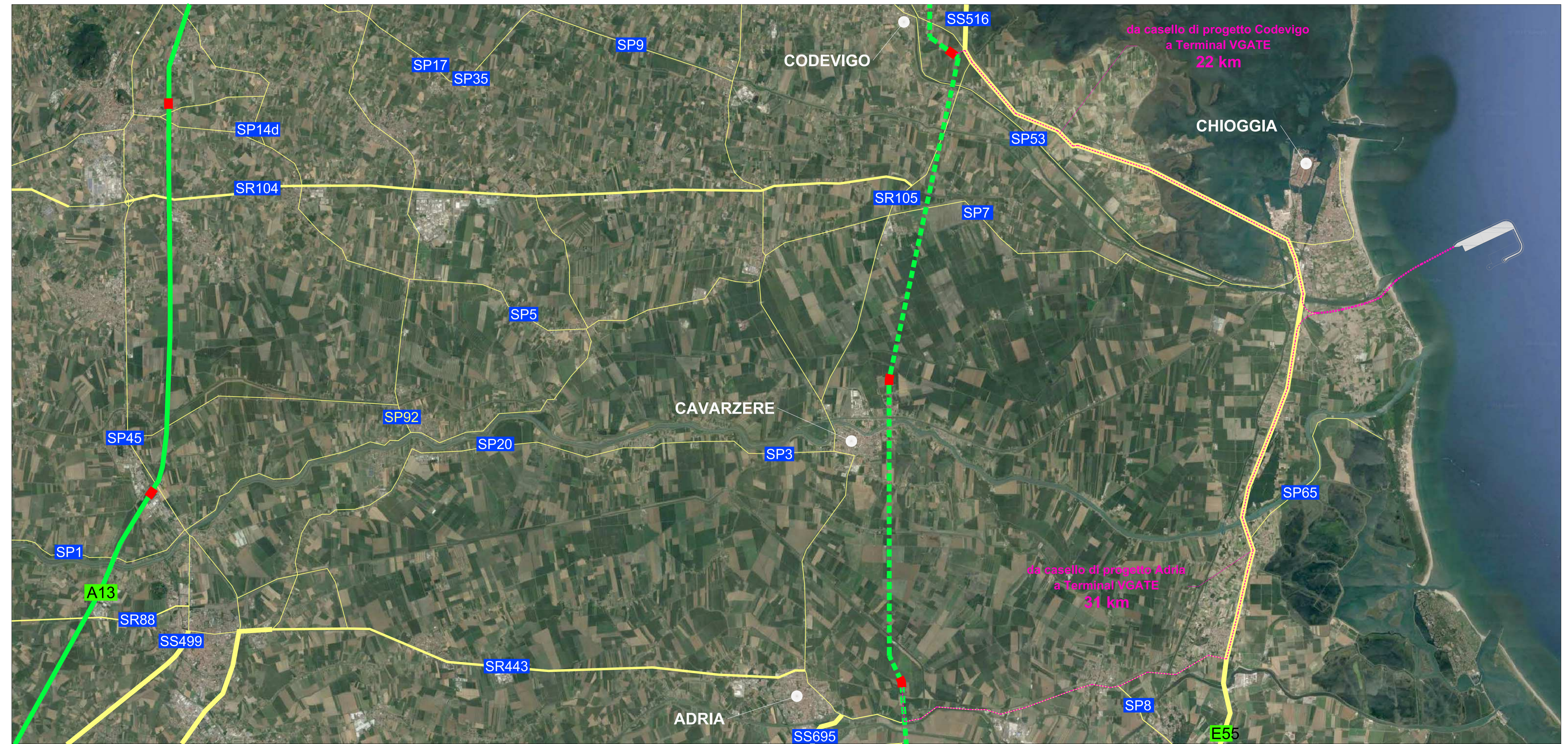
PLANIMETRIA GENERALE viabilità stradale - Scala 1:50.000
