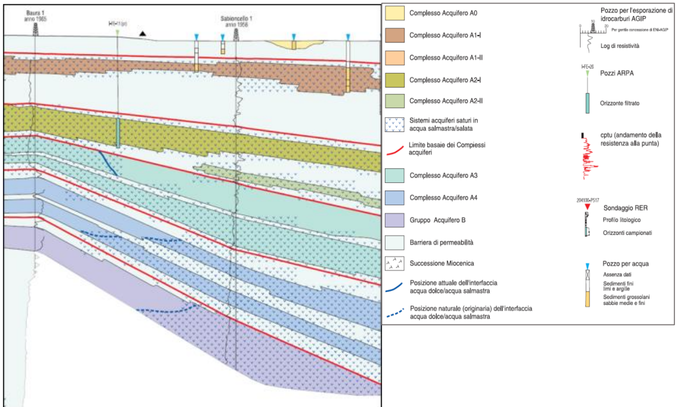
Figura 2.17 - Sezione Idrostratigrafica del sottosuolo e suddivisione in Gruppi Acquiferi (fonte: Regione Emilia Romagna, sito web). Il triangolo nero riporta l'ubicazione dell'area oggetto di studio.
