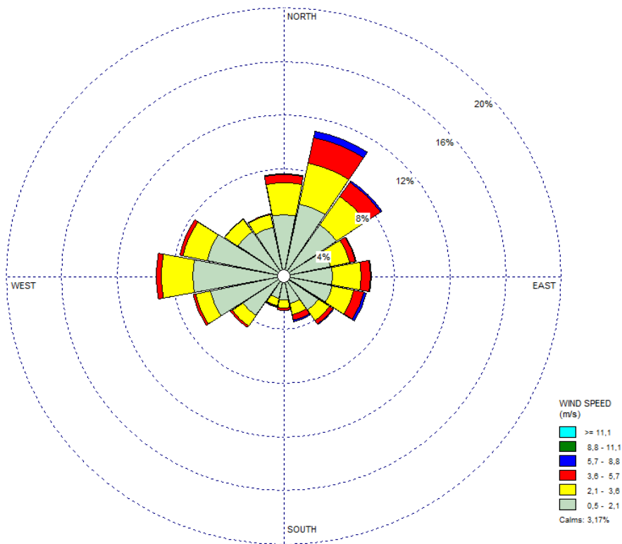
Figura 2.10 - Rosa dei venti per l'anno 2013 relativa alla stazione di Malborghetto di Boara
