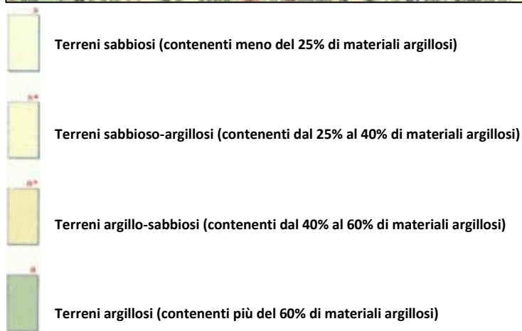
Figura 2.22 - Stralcio della Carta Geologica d'Italia, Foglio 76 Ferrara, scala 1:100.000 (fonte: ISPRA Ambiente, sito web)
