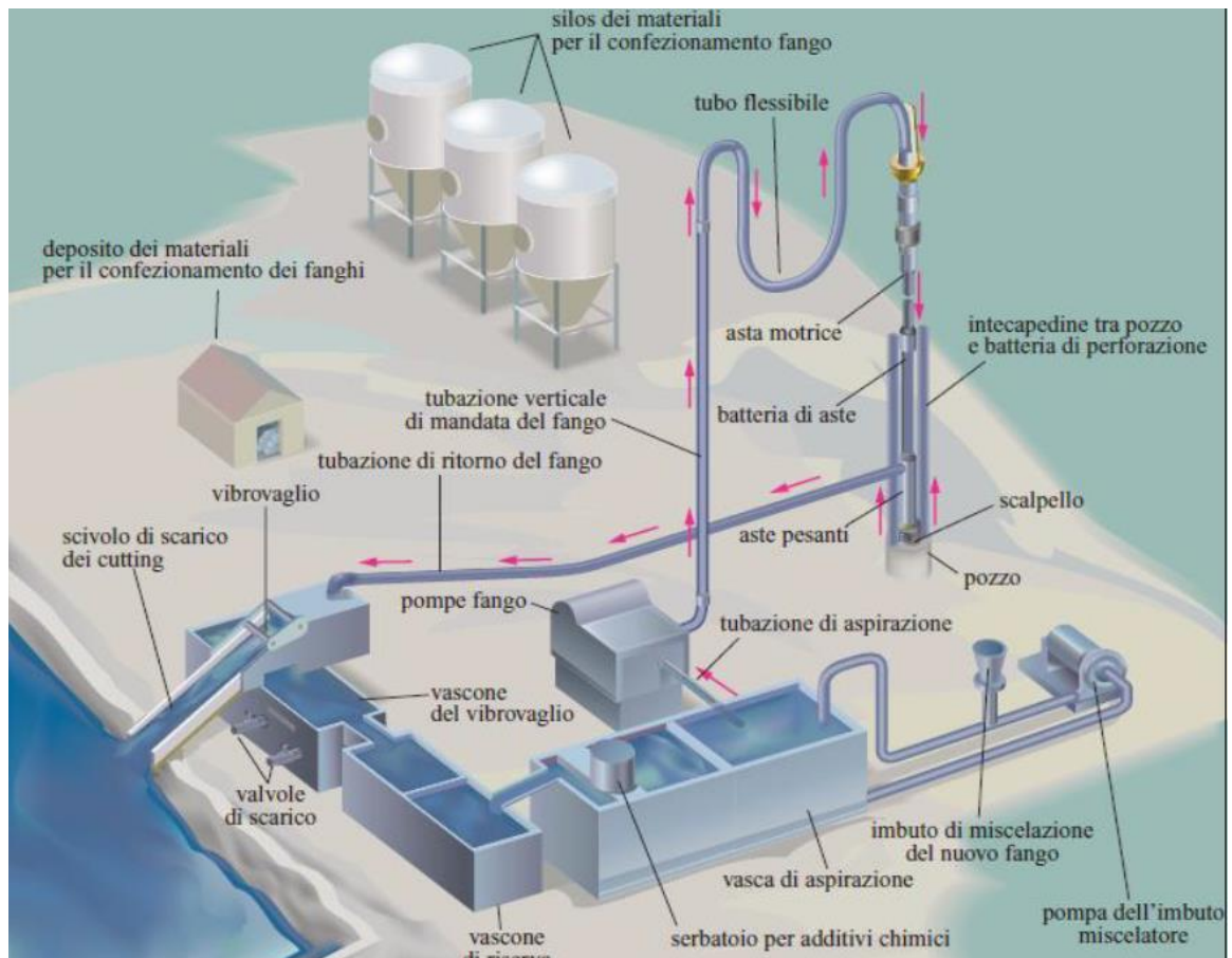
Figura 2.7 - Circuito del fango in impianto
