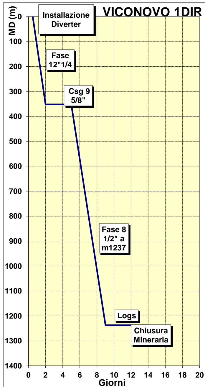
Figura 2.8 - Diagramma delle fasi di perforazione previste
