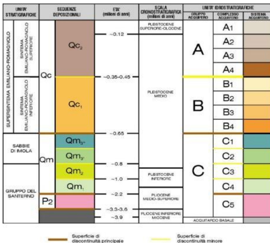
Figura 2.16 - Depositi della pianura suddivisi in tre unità stratigrafiche: Gruppi Acquiferi A, B e C (fonte: Regione Emilia Romagna, http://ambiente.regione.emilia-romagna.it/geologia/temi/acque/idrogeologia-della-pianura-emiliano-romagnola )
