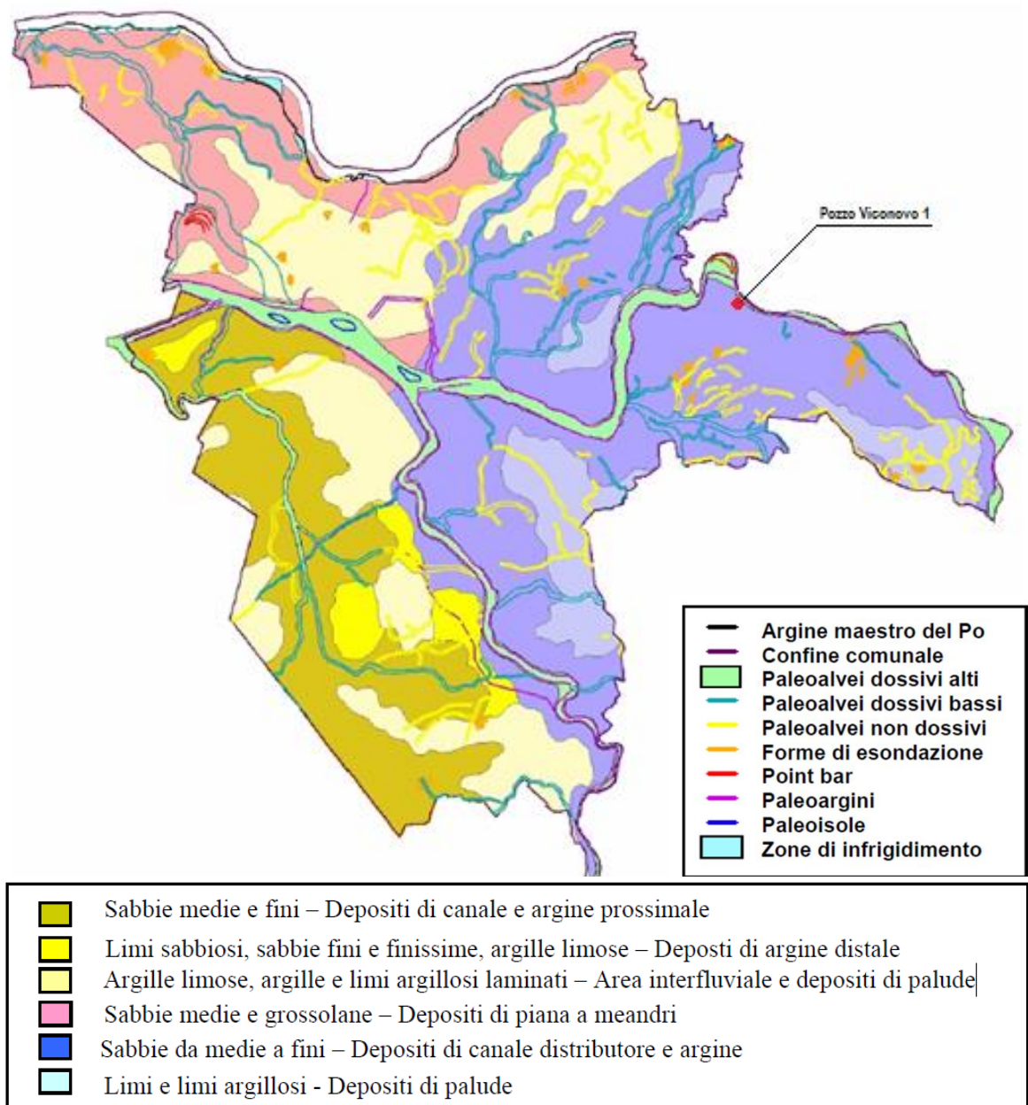
Figura 2.23 – Stralcio della Carta Geologica Provinciale di Pianura (fonte: Comune di Ferrara, sito web )
