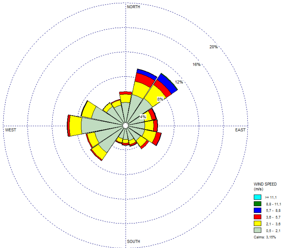
Figura 2.9 - Rosa dei venti per l'anno 2012 relativa alla stazione di Malborghetto di Boara
